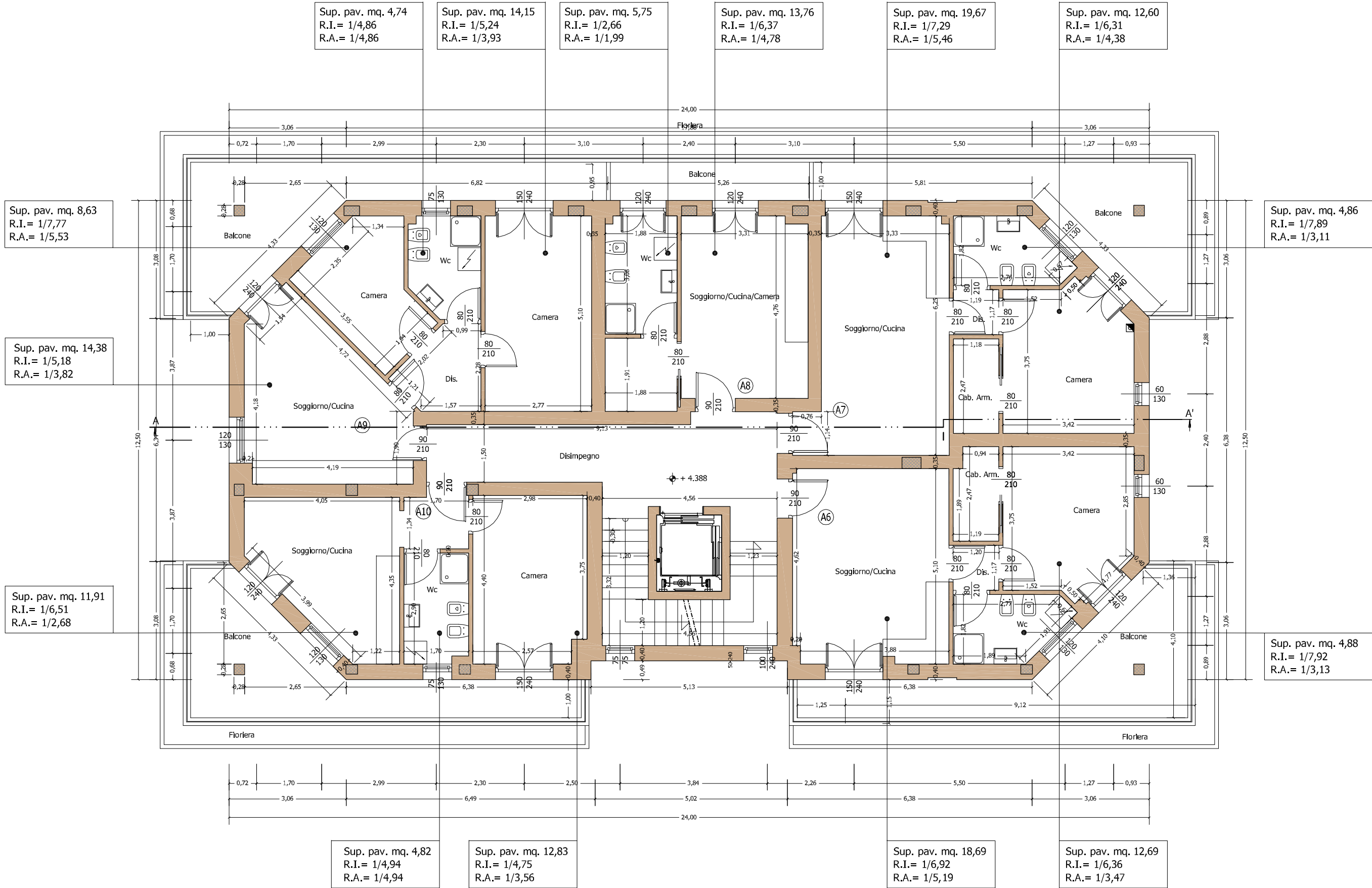
PIANTA PIANO PRIMO_progetto_scala 1:100
