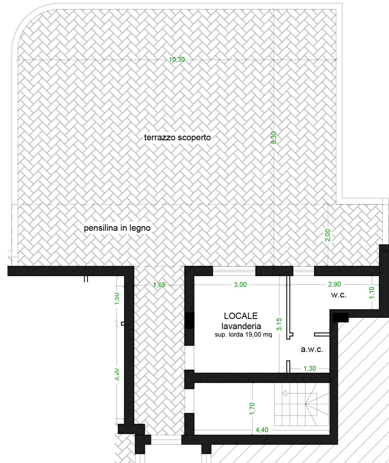
PIANTA PIANO QUINTO
