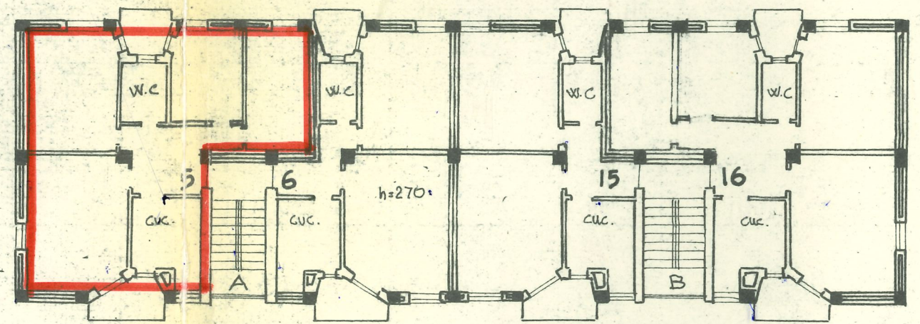
FOGLIO 51 NUMERO 158 SUBALTERNO 5 17 A CASA POPOLARE FALSO ENZO PIANTA PIANO SECONDO
