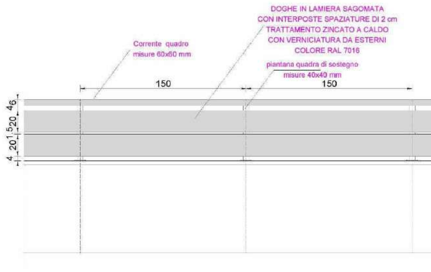
PARTICOLARE COSTRUTTIVO TIPO
