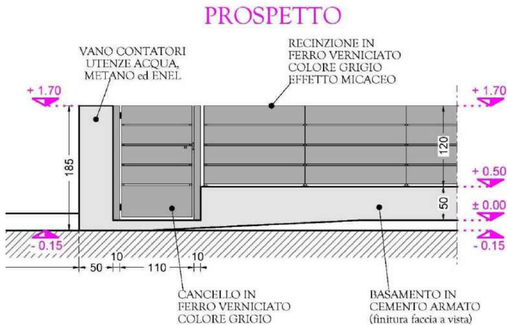
PARTICOLARE COSTRUTTIVO TIPO
