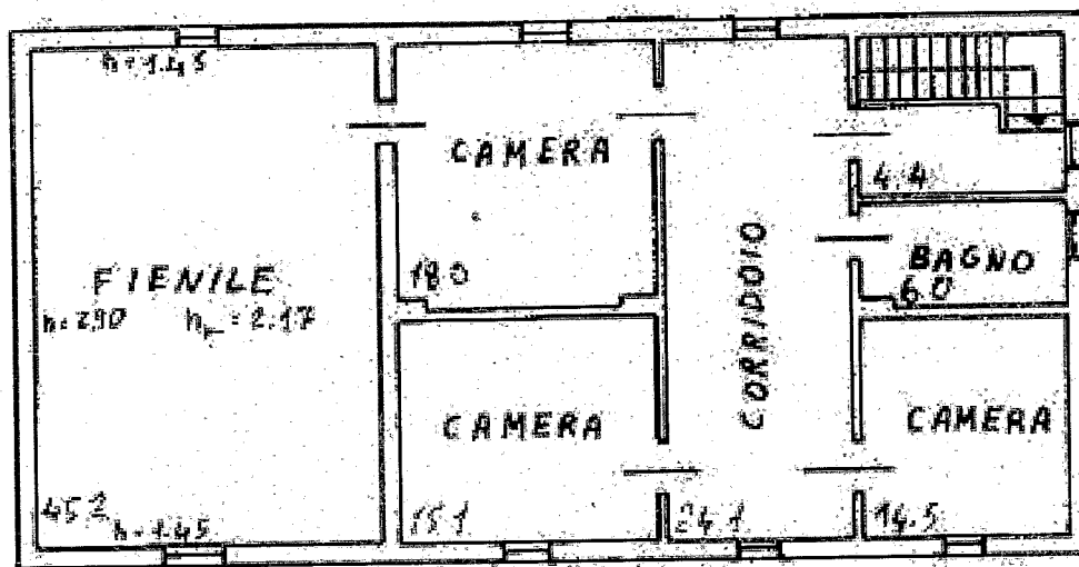
PIANO PRIMO H = 240
