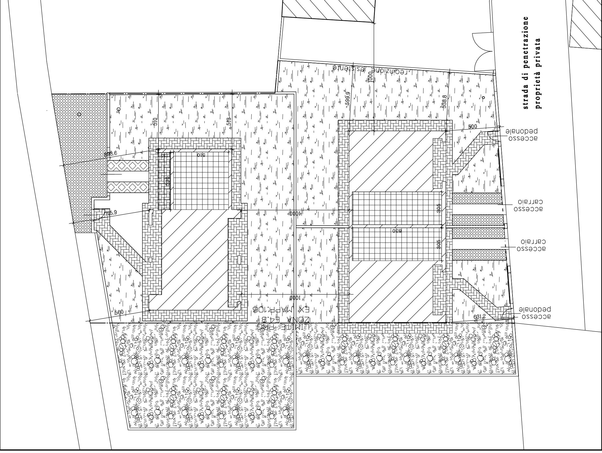
PIANTA 1:200
