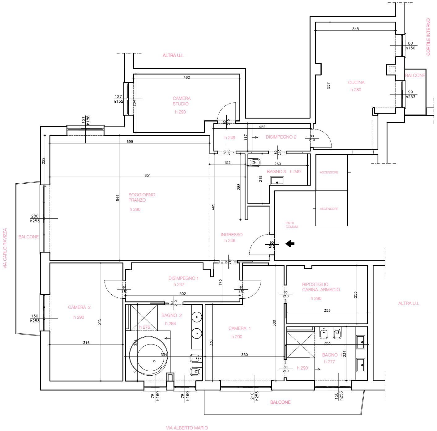
PIANTA UNITA' IMMOBILIARE - PIANO QUARTO
