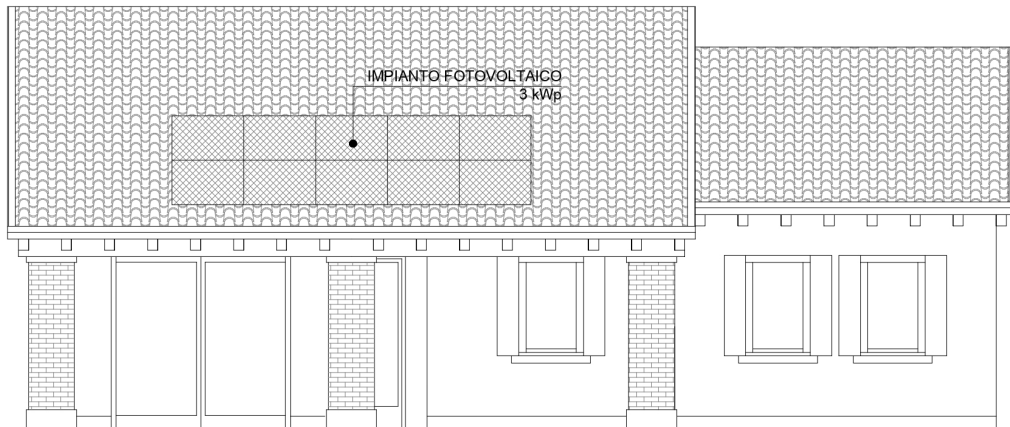
PROSPETTO SUD
