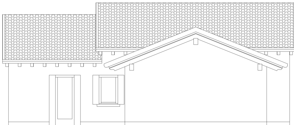
PROSPETTO NORD
