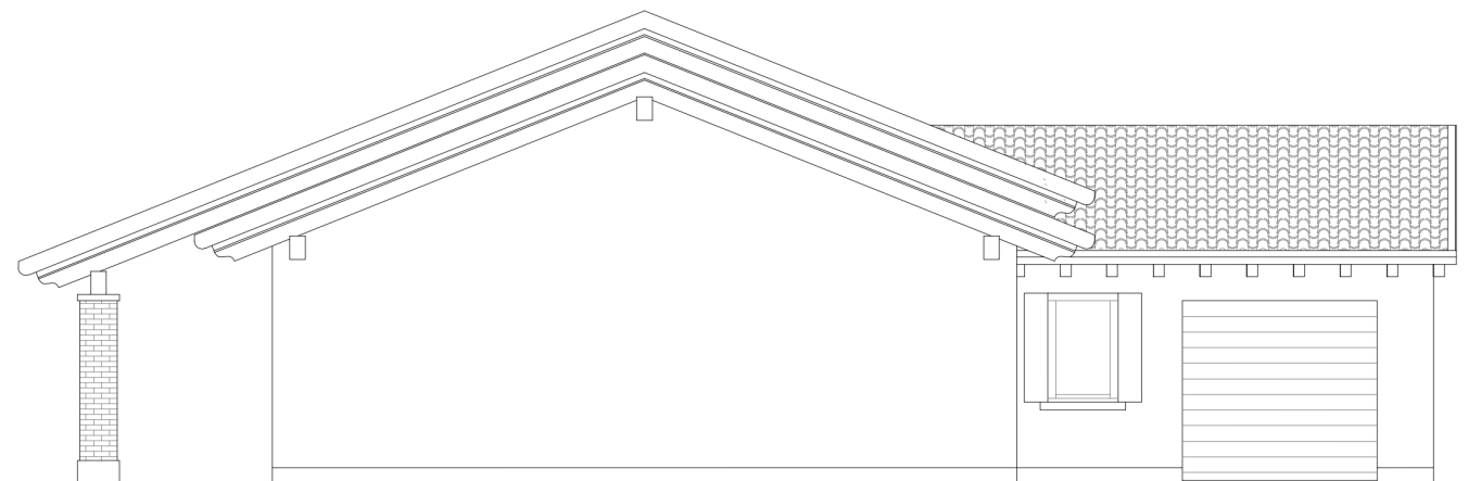
PROSPETTO EST
