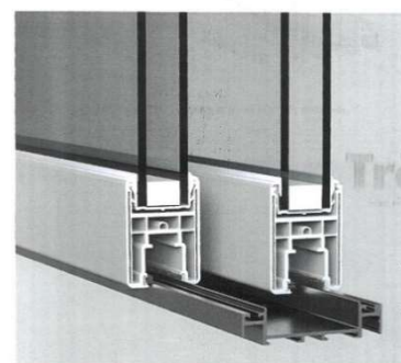
Particolare scorrevole parallelo portafinestra con soglia in alluminio
