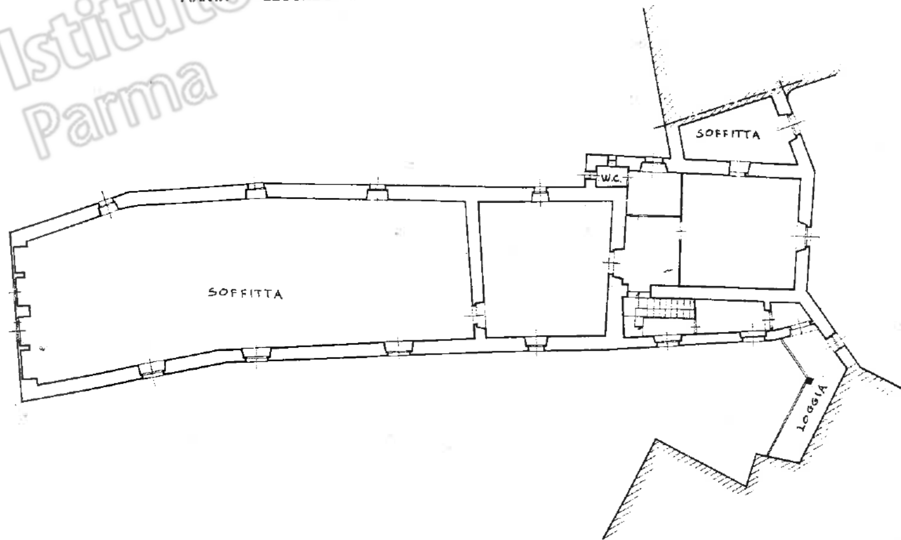
PIANTA SECONDO PIANO
