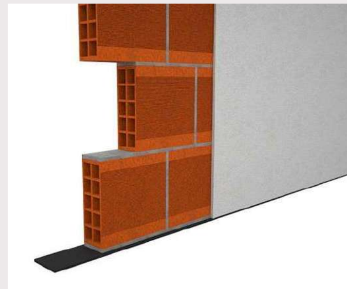
Figura 18 – Fascia tagliamuro
