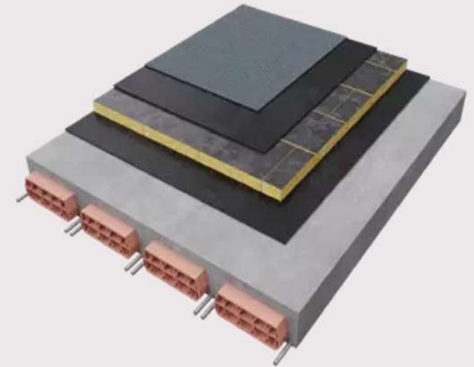
Figura 16 – Pacchetto copertura
