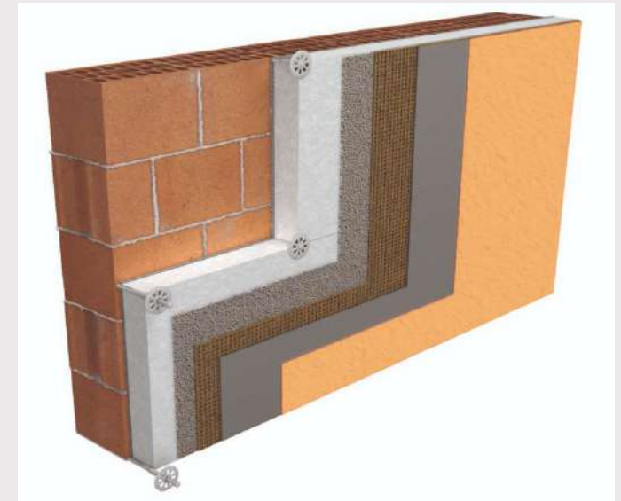
Figura 12 – Esempio cappotto
