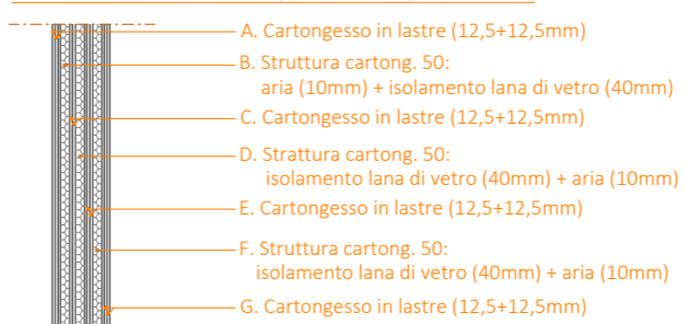
PARTICOLARE 3: Divisorio tra appartamenti. Spessore 25 cm
