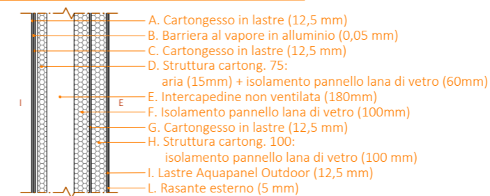
PARTICOLARE 1.1: Pareti perimetrali. Spessore 51 cm
