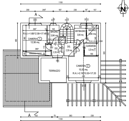
PIANO PRIMO quota +3,40 m
