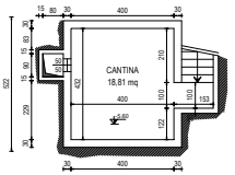
PIANO SECONDO INTERRATO quota -4,30
