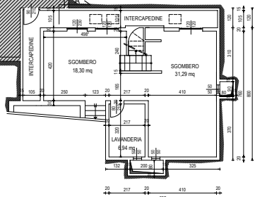
PIANO PRIMO INTERRATO quota -2,80 m
