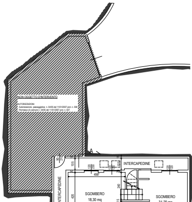
PIANO SECONDO INTERRATO quota -4,30
