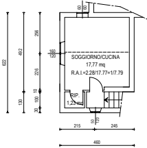
PIANO RIALZATO quota +1,50 m
