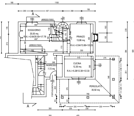
PIANO TERRA quota ± 0,00 m
