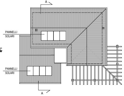
PIANTA TETTO
