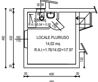
PIANO PRIMO INTERRATO quota -1,30 m
