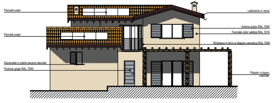
PROSPETTO SUD
