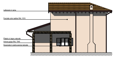
PROSPETTO EST
