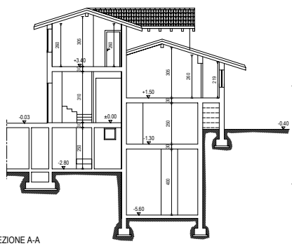
SEZIONE A-A
