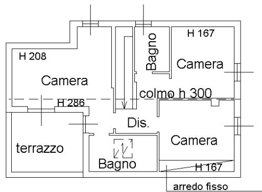
PIANO SOTTOTETTO
