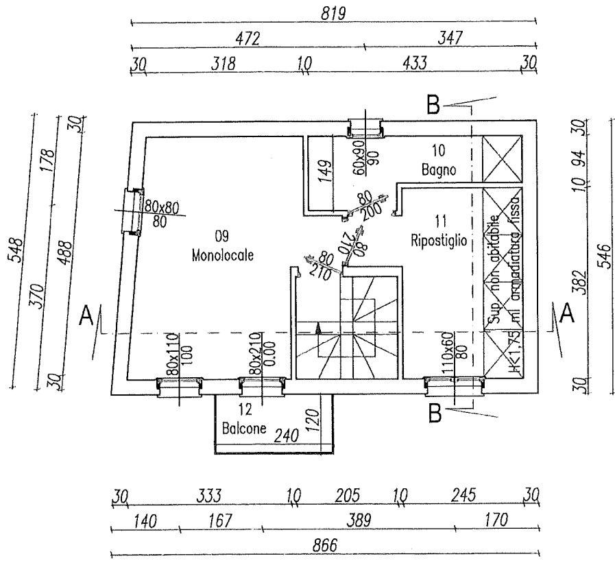
PIANO SECONDO
