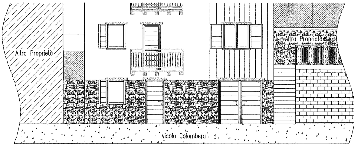
PROSPETTO EST
