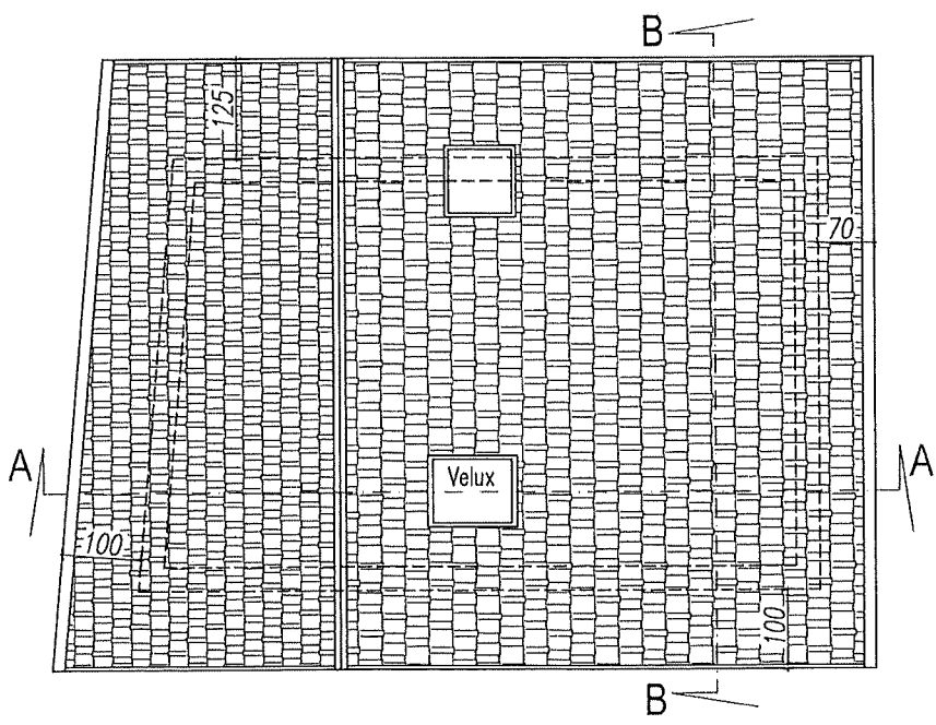
PIANTA COPERTURA
