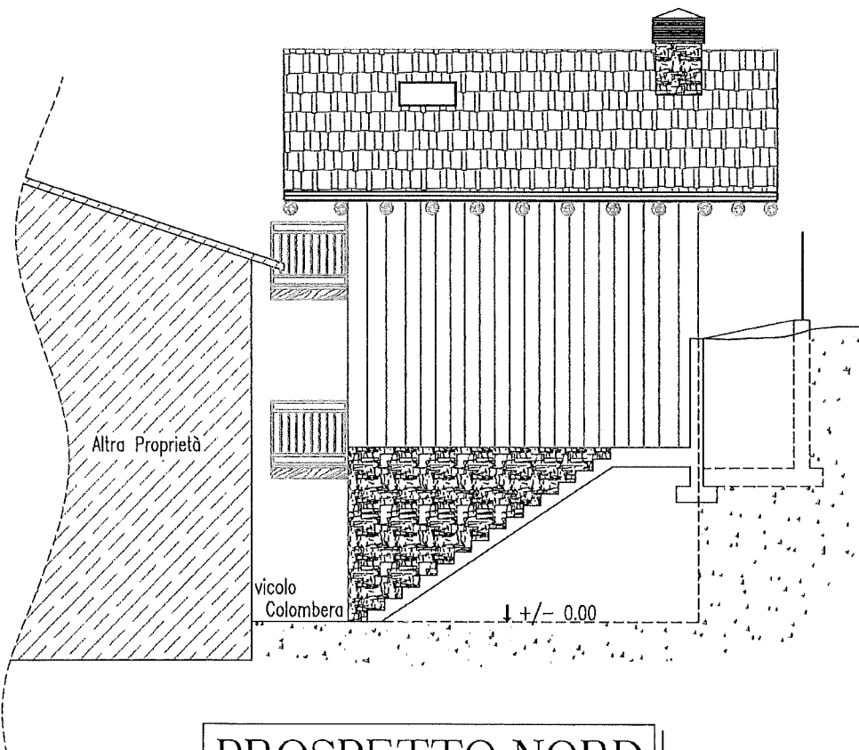
PROSPETTO NORD
