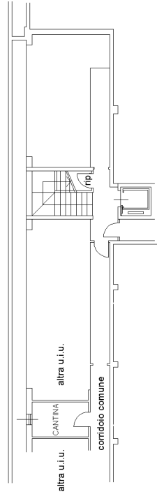
PIANO PRIMO SOTTOSTRADA H= 2,47
