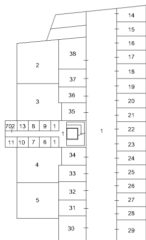
PIANO PRIMO INTERRATO
