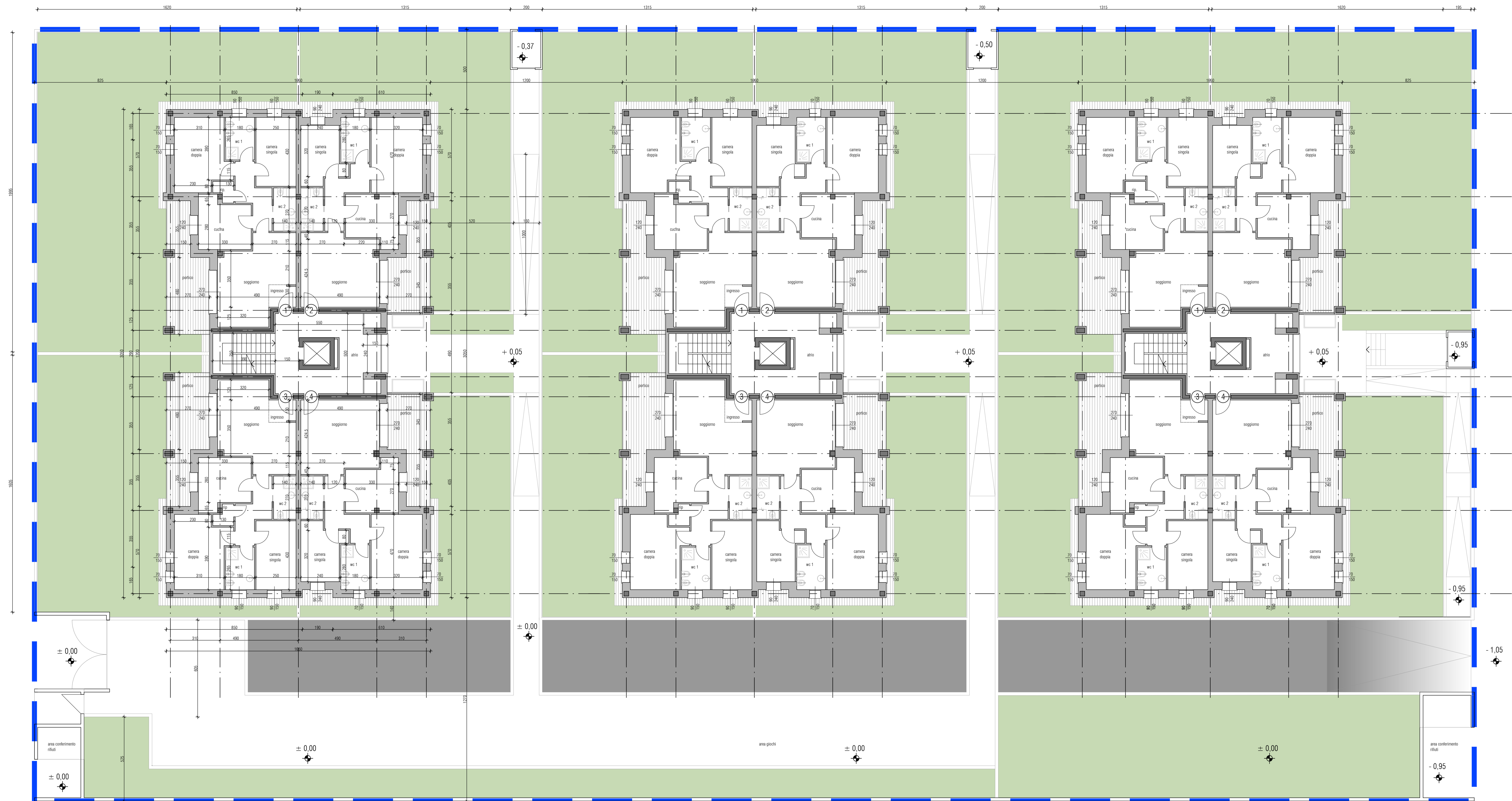
PIANTA PIANO TERRA - SCALA 1/100
