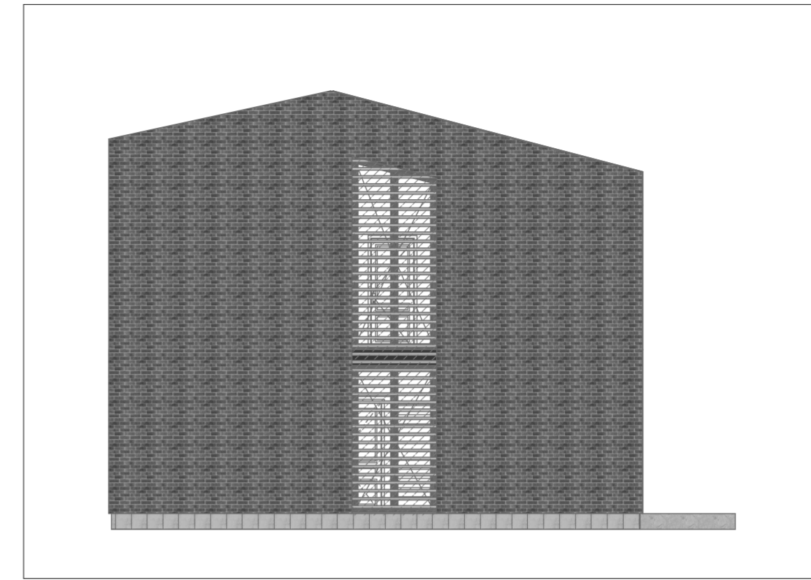
Alzato Est (2)
