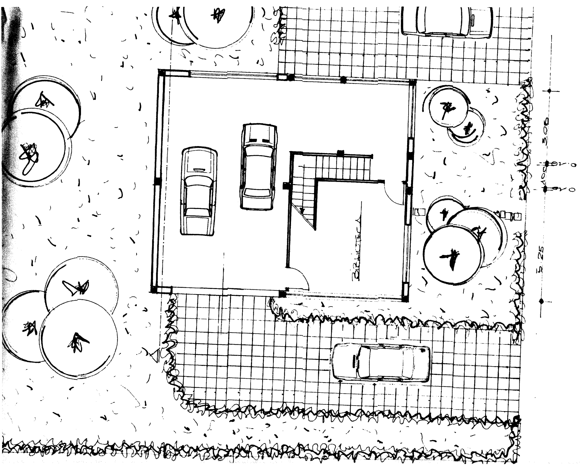
PIANTA PIANO SCANTINATO
