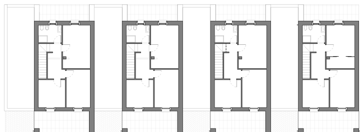
2 Planimetria piano primo
