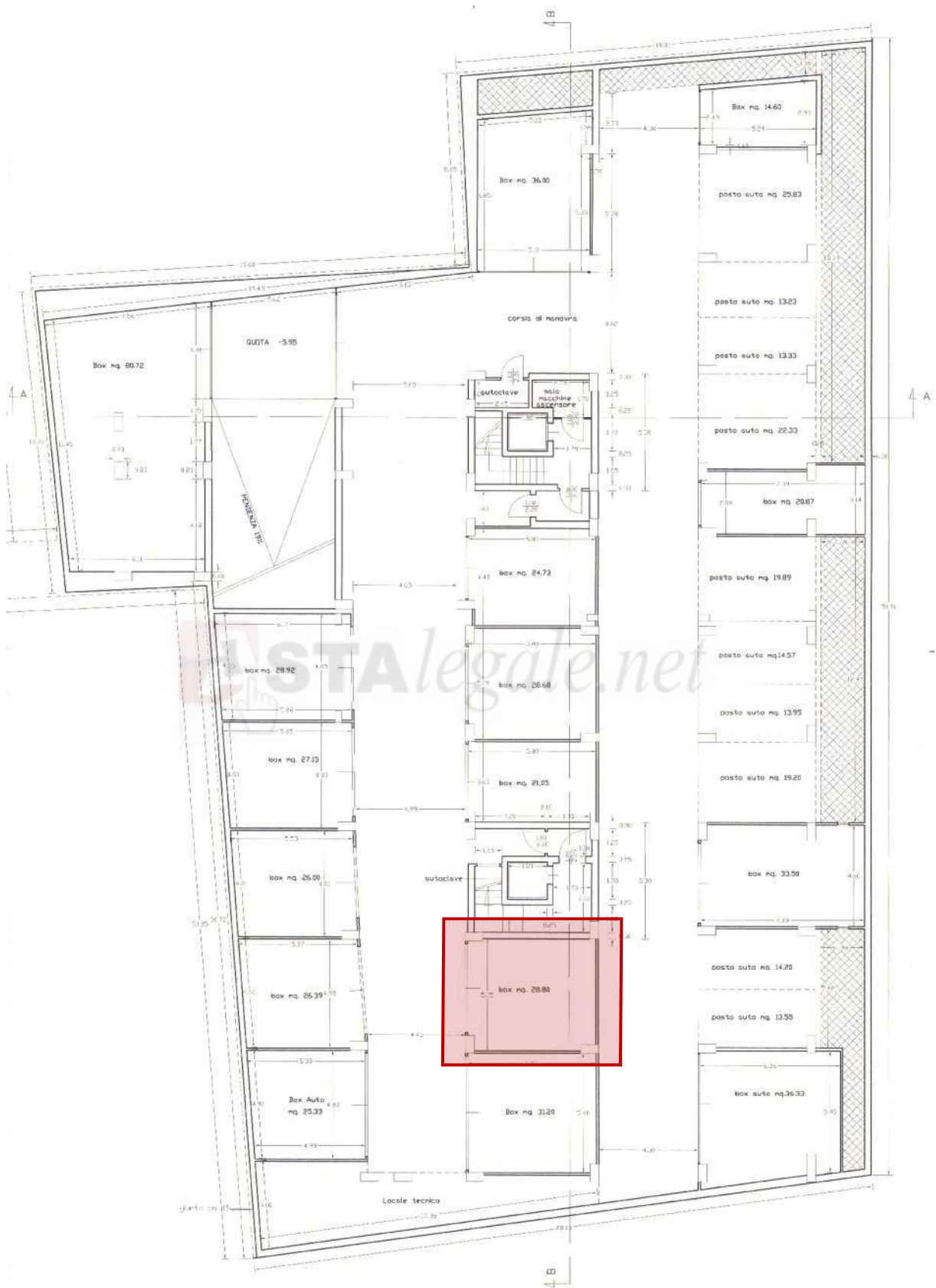
Figura n. 2.12 : Tav. 01 - Pianta Piano Sottostrada 2° livello Quota -5.80 m (C.E.73/2011) con indicaz. del Sub 50
