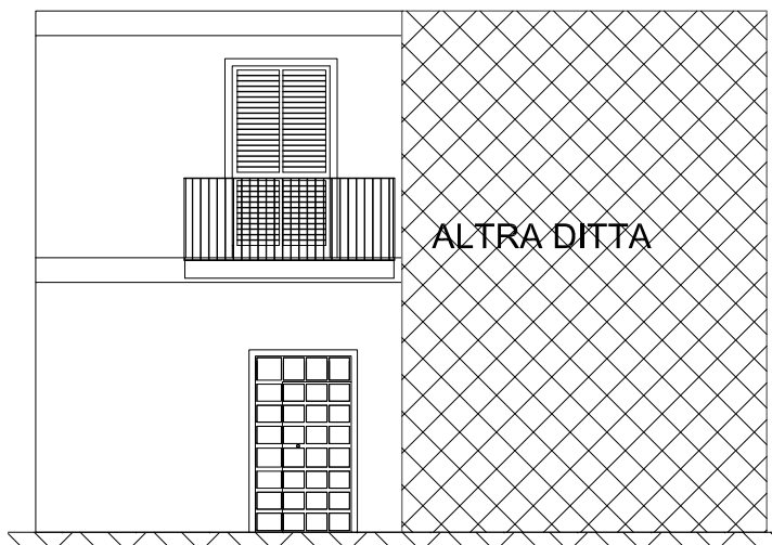
PROSPETTO SU VIA PRINCIPESSA DELIELLA
