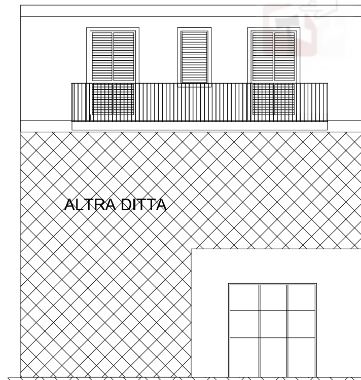
PROSPETTO SU VIA SANT'ELIA
