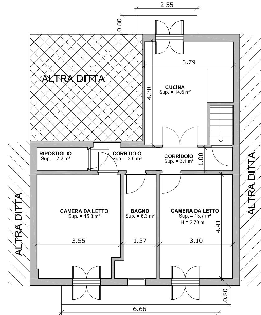
SCHIZZO PIANTA PIANO PRIMO
