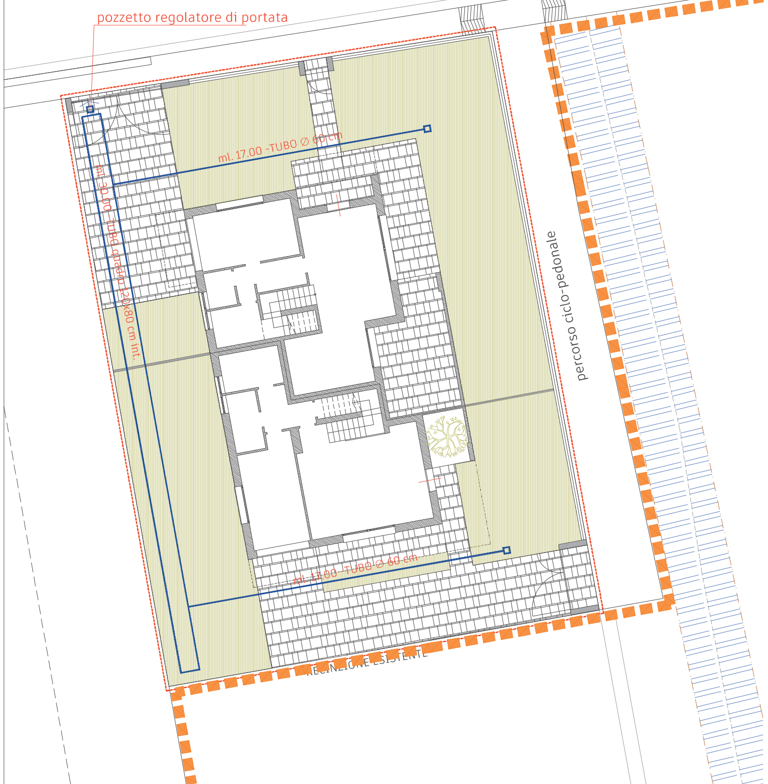
PLANIMETRIA GENERALE DIMOSTRAZIONE INVARIANZA IDRAULICA
