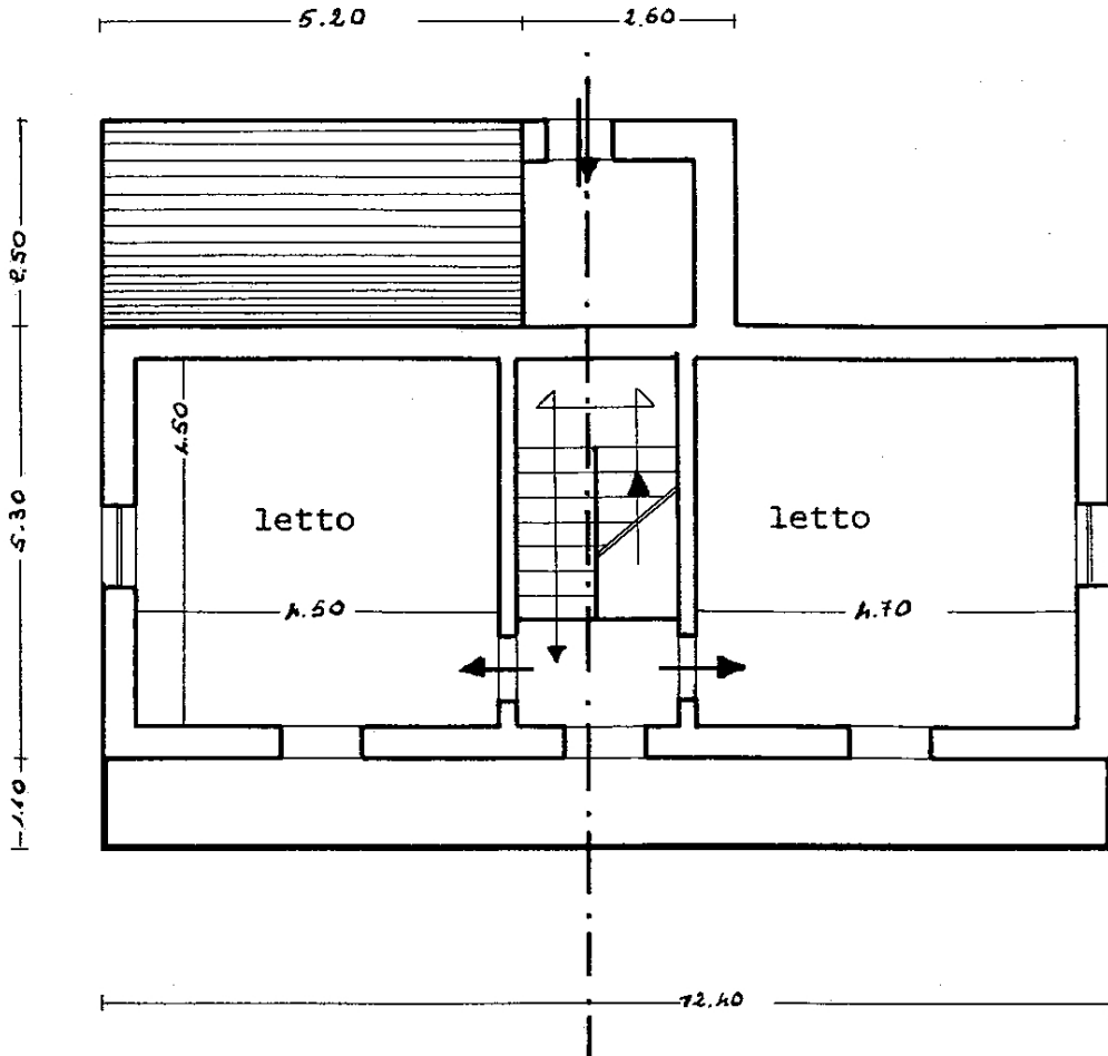
Pianta piano elevato
