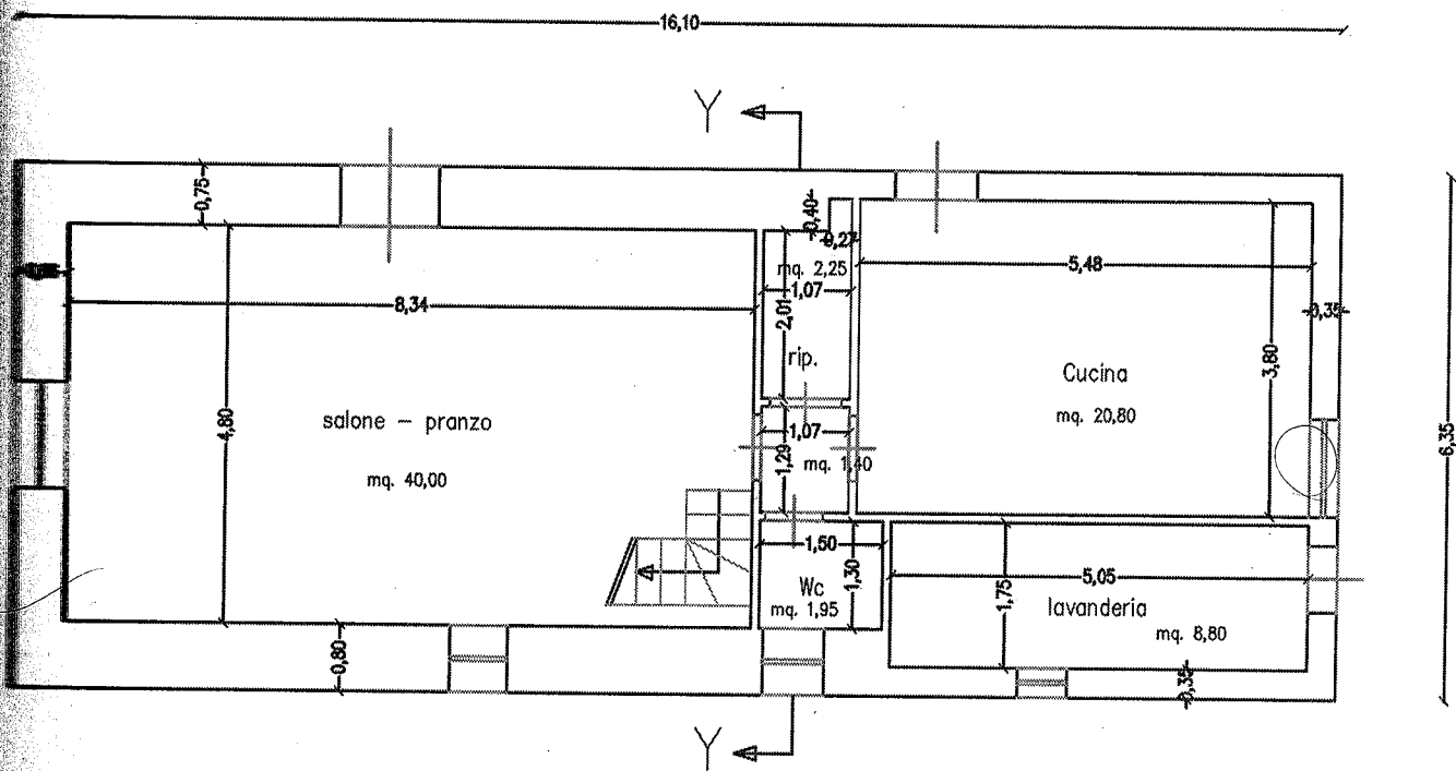
PIANTA PIANO TERRA ATTUALE
