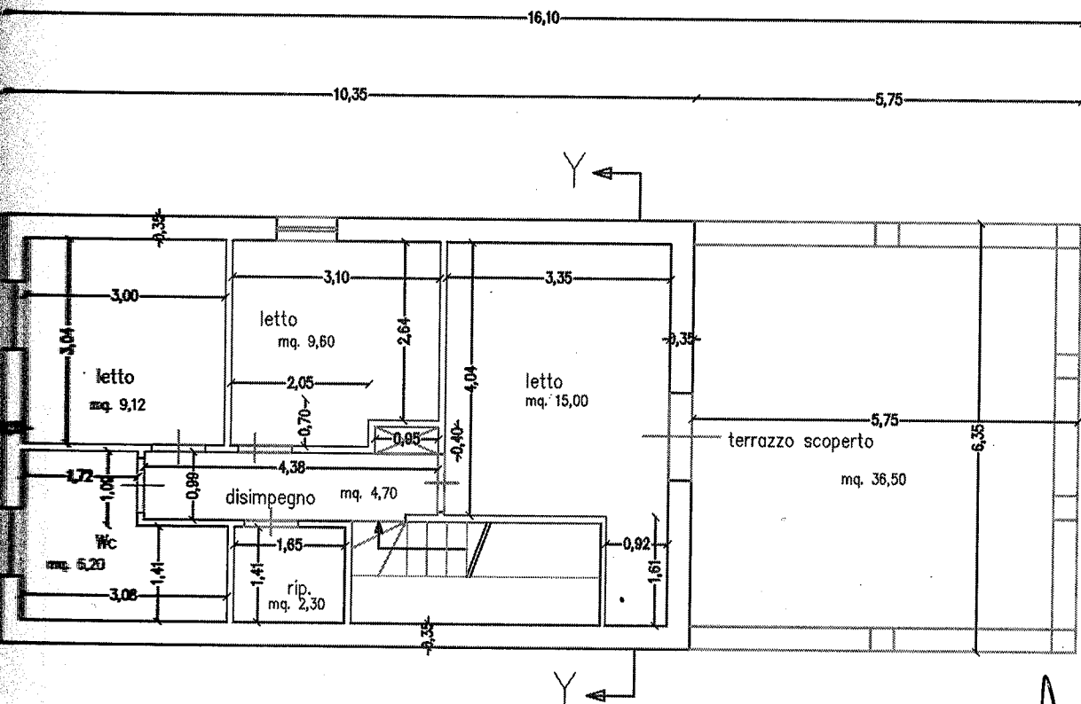
PIANTA PIANO PRIMO ATTUALE
