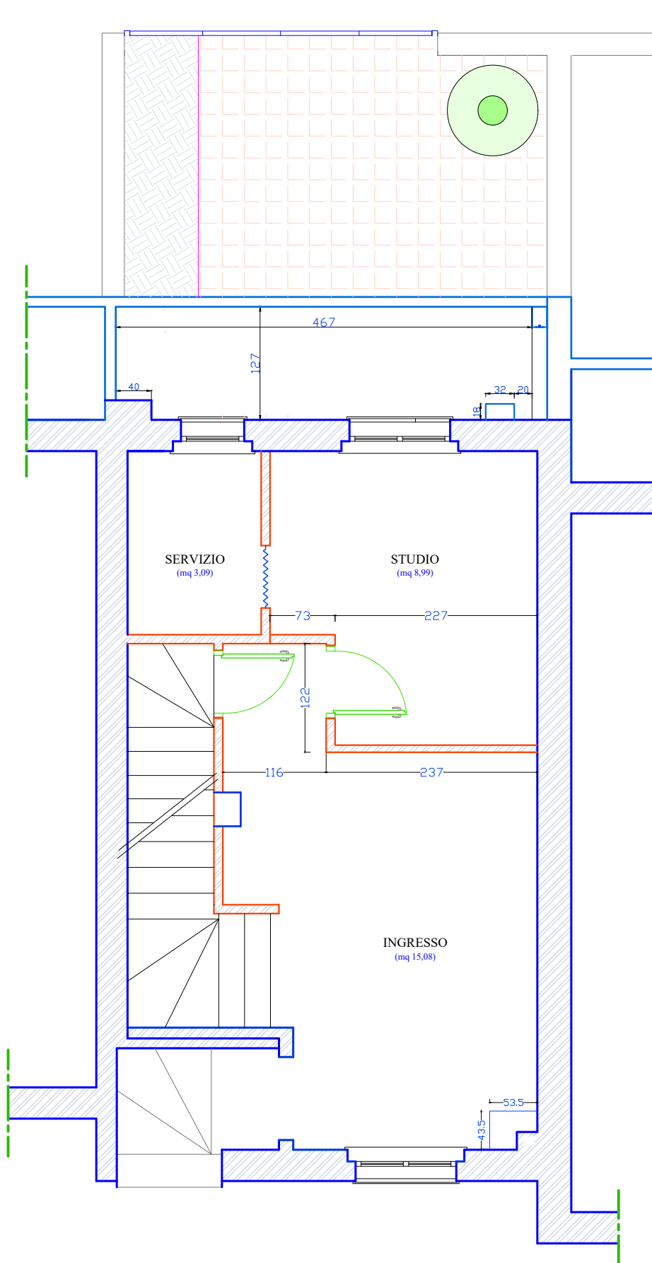
PIANO RIALZATO (mq 27,16)
