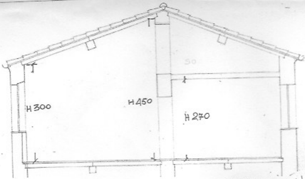
SEZIONE AA'
