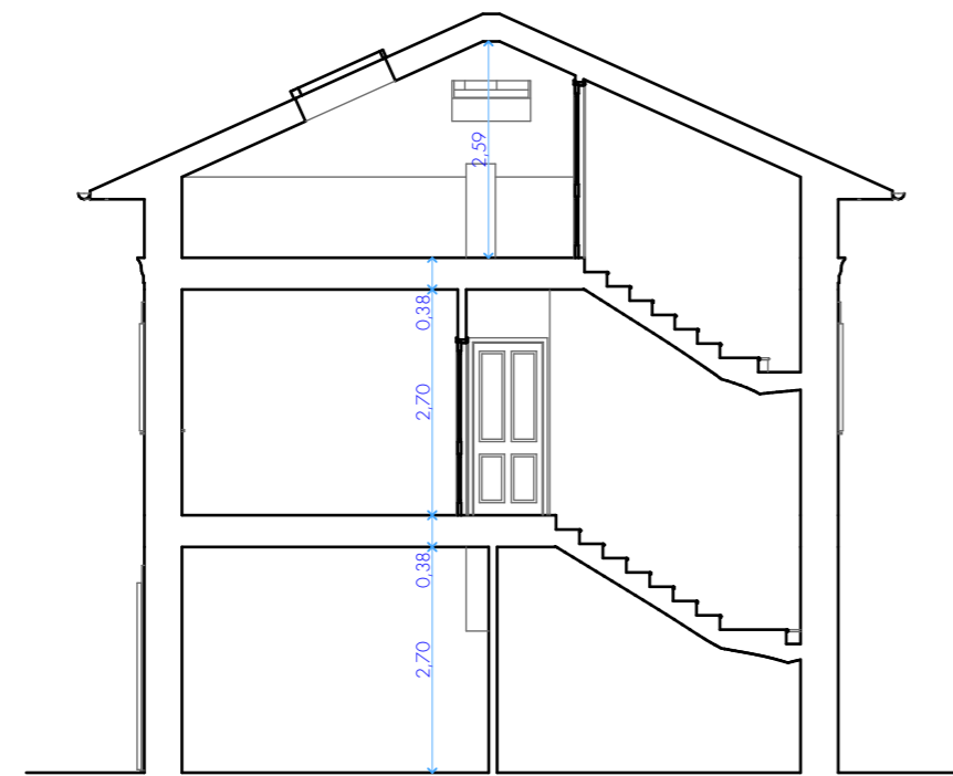
S2 Sezione 2 1:100
