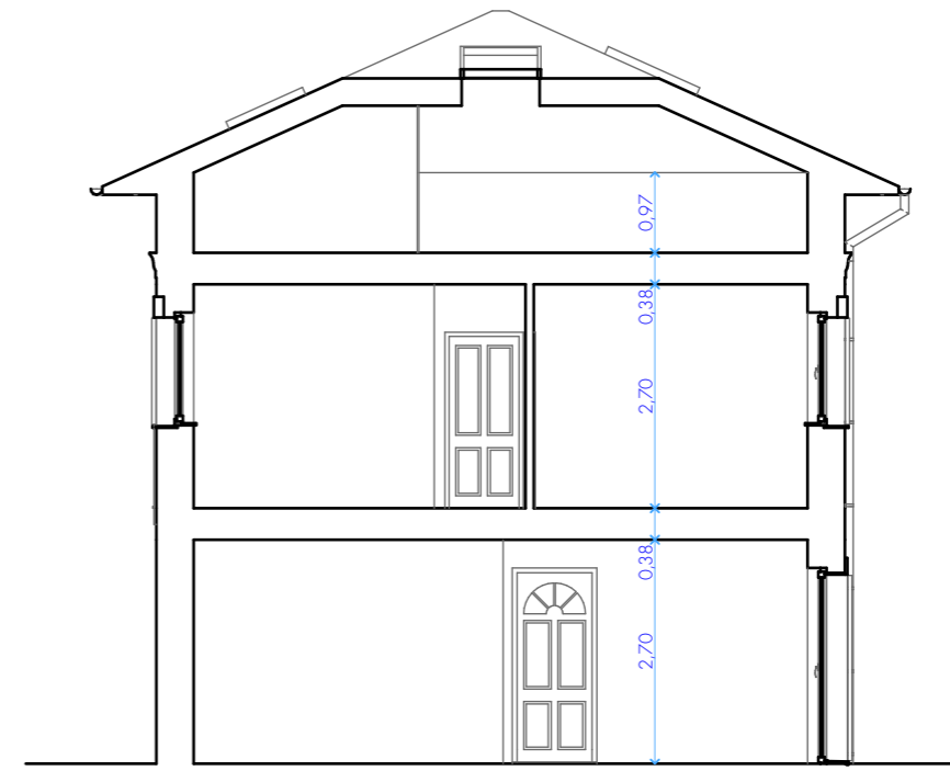
S3 Sezione 3 1:100
