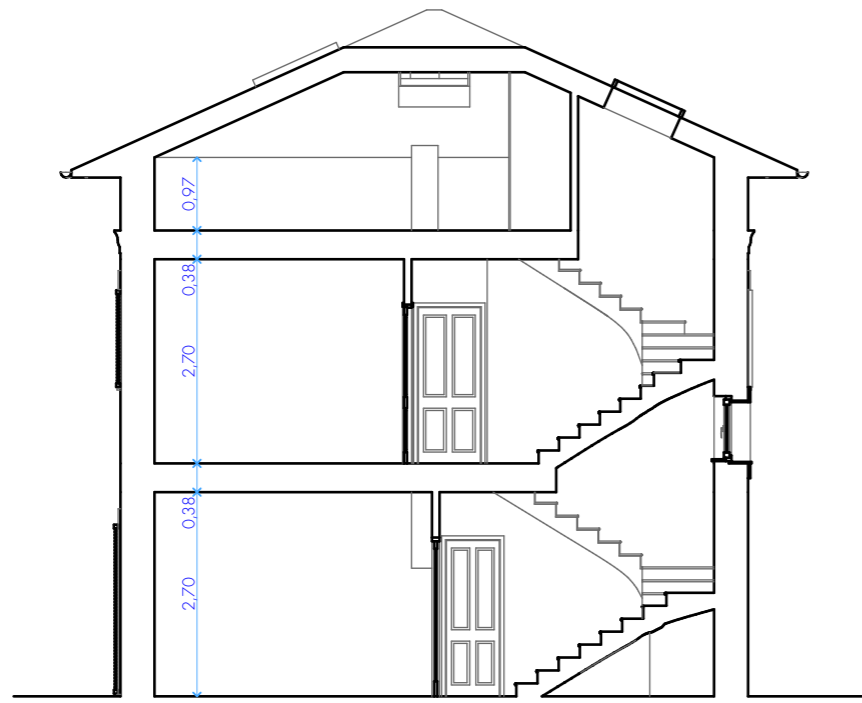
S1 Sezione 1 1:100
