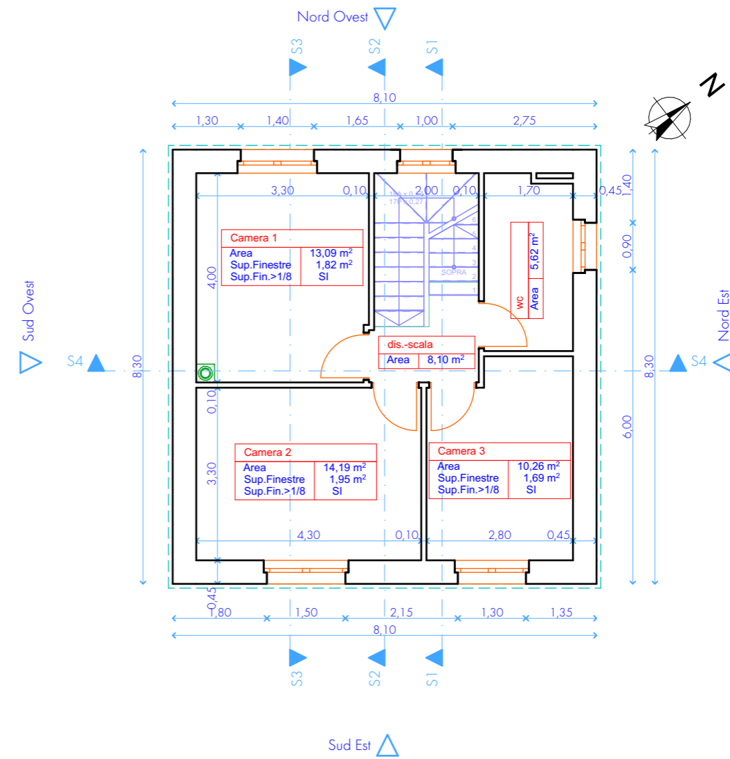
1. Piano Primo 1:100
