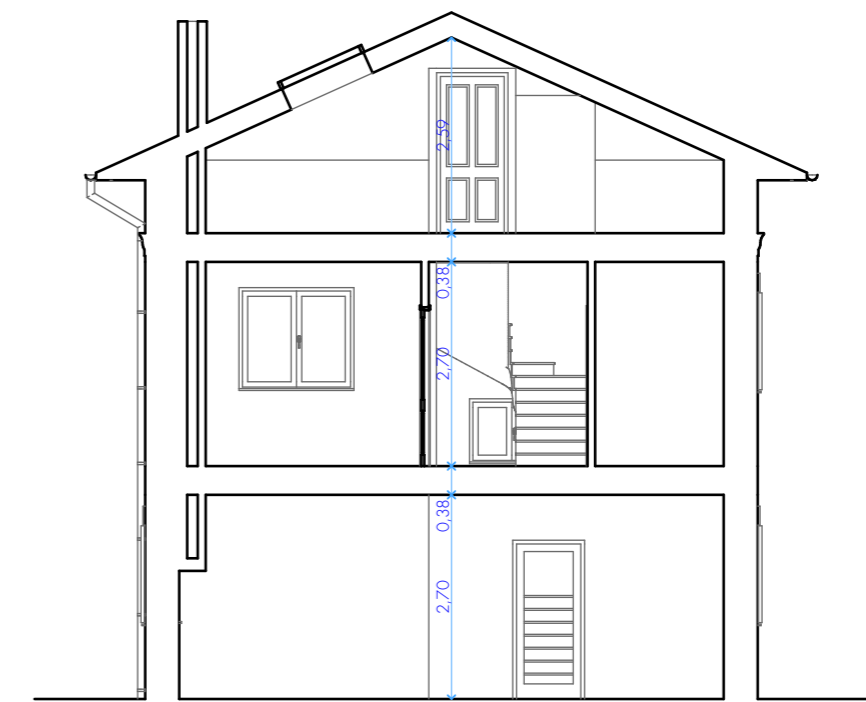
S4 Sezione 4 1:100
