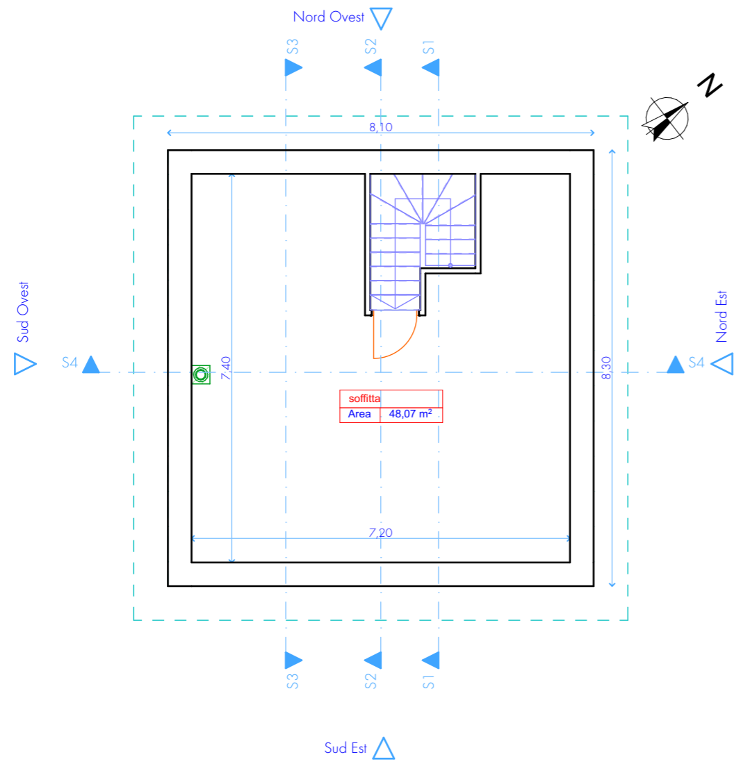
2. Piano Sottotetto 1:100
