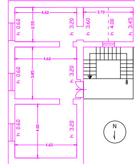
Pianta Sottotetto
