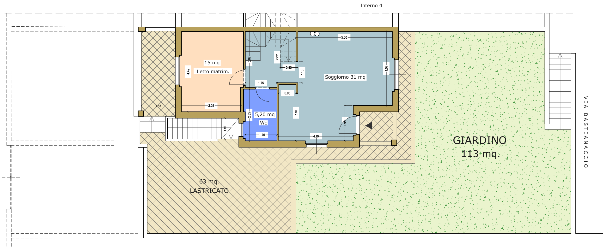
Pianta piano terra 1:100
