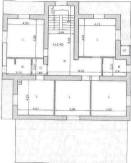
Piano Primo scala 1 : 100
