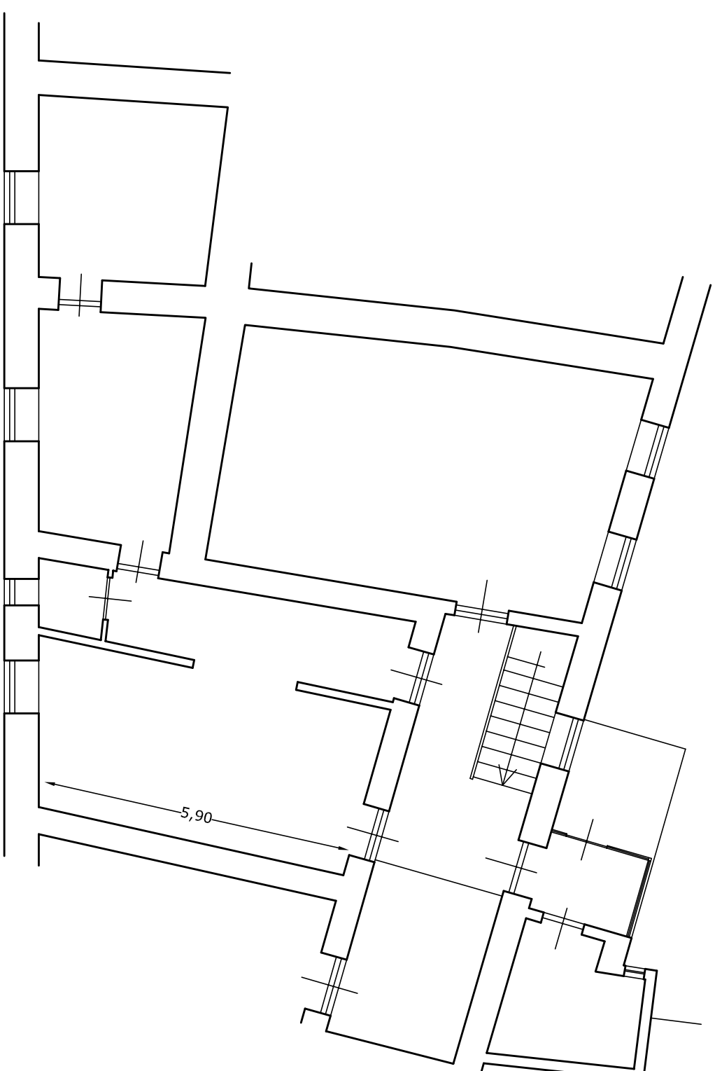
Piano Primo h = mt 2,80
