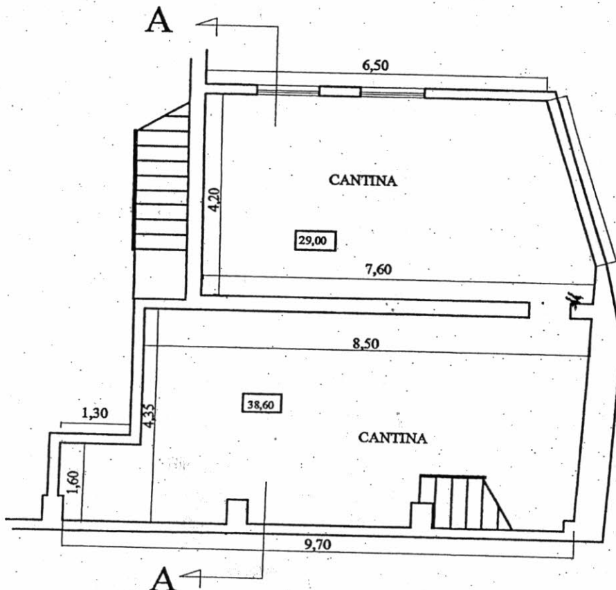
PIANTA PIANO SECONDO INTERRATO H.m. 3,48
