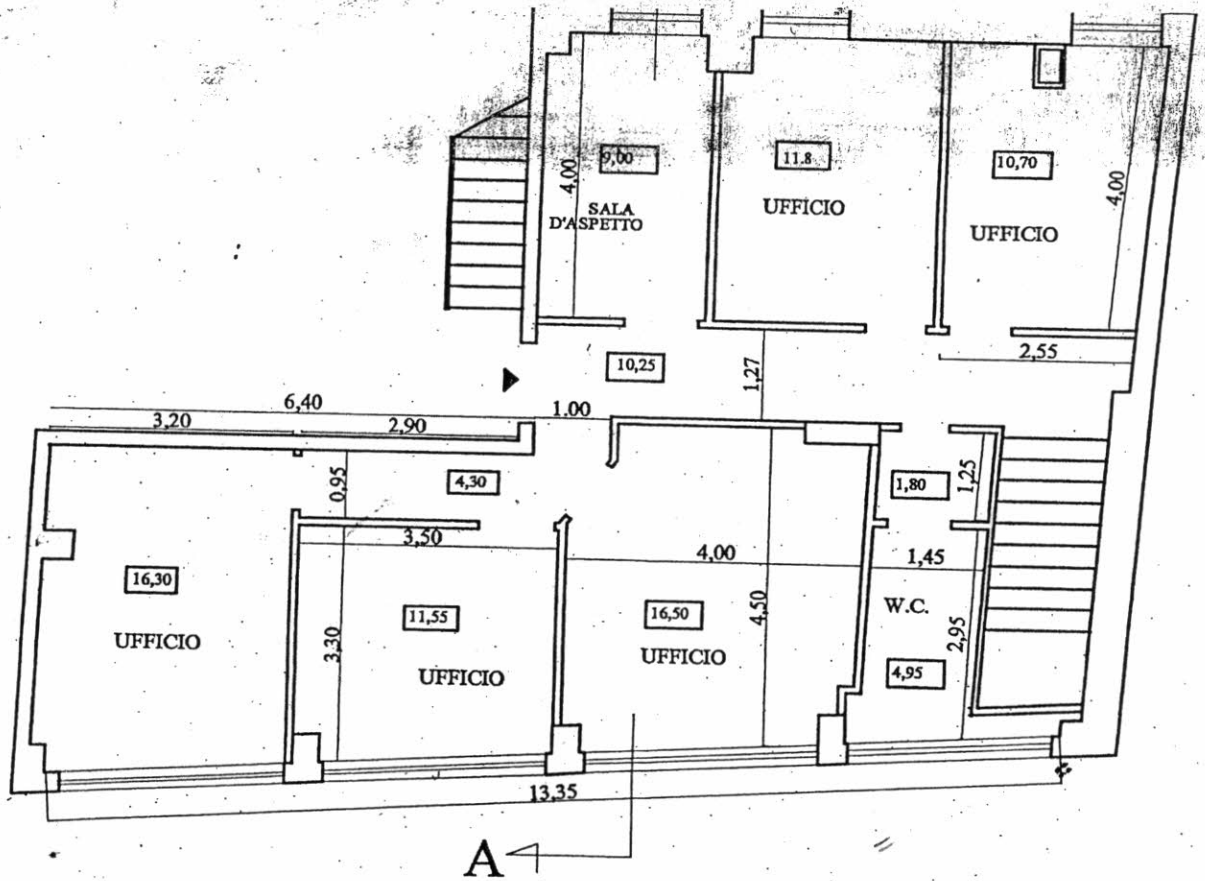
PIANTA PIANO PRIMO INTERRATO H.M.3,00
