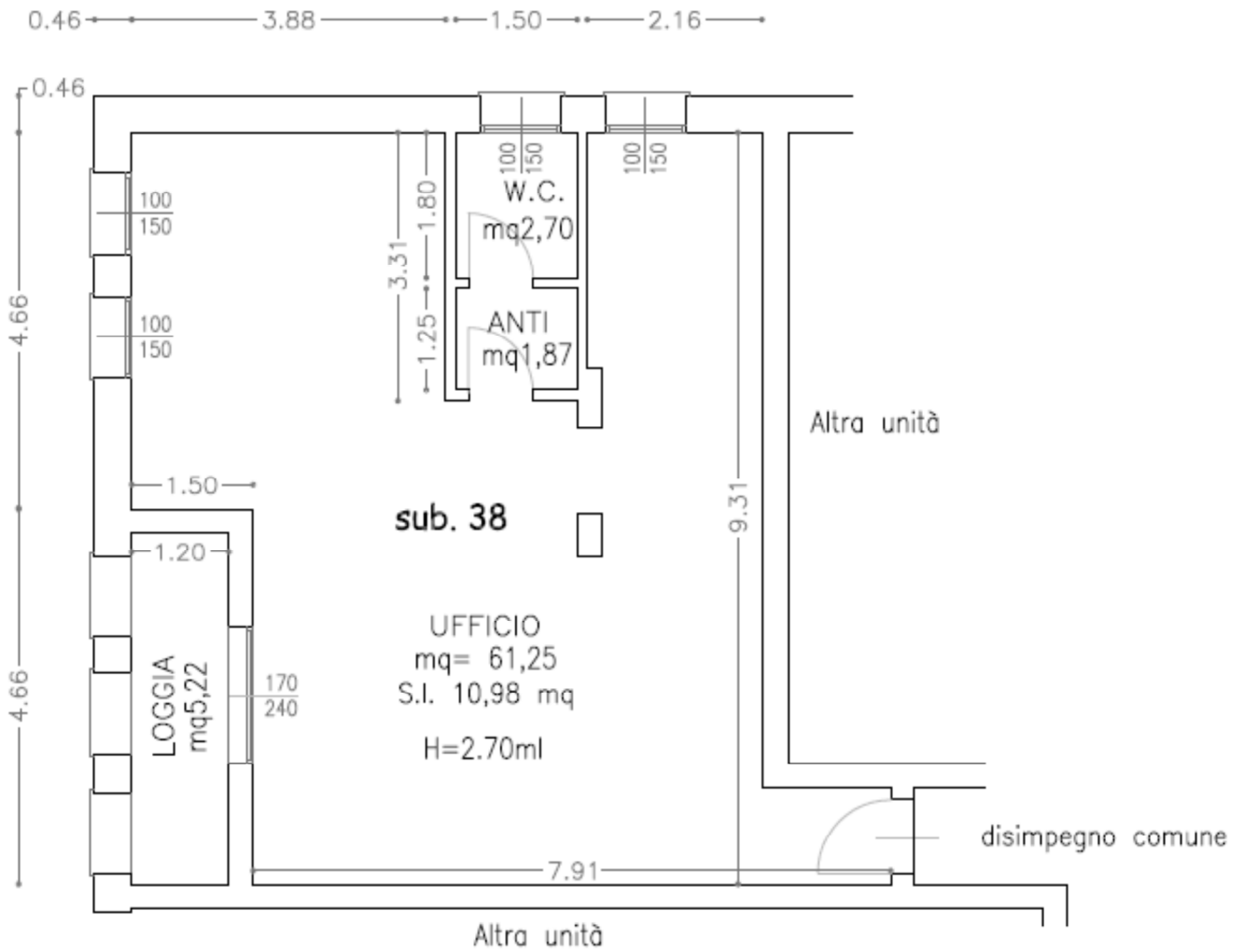
PIANTA PIANO SECONDO h=2.70ml Scala 1:100
