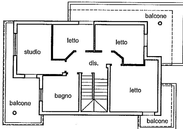
Piano primo
