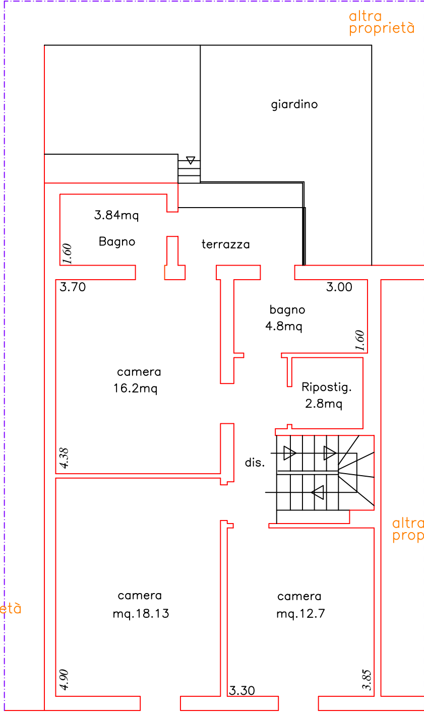
PIANO PRIMO
