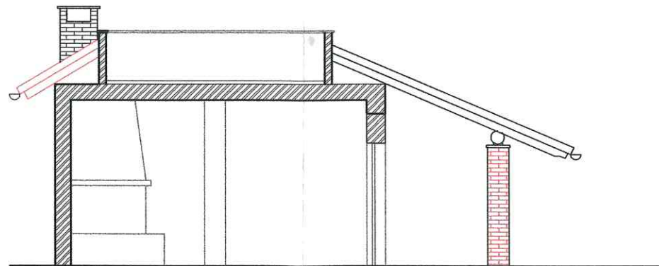
Sezione
