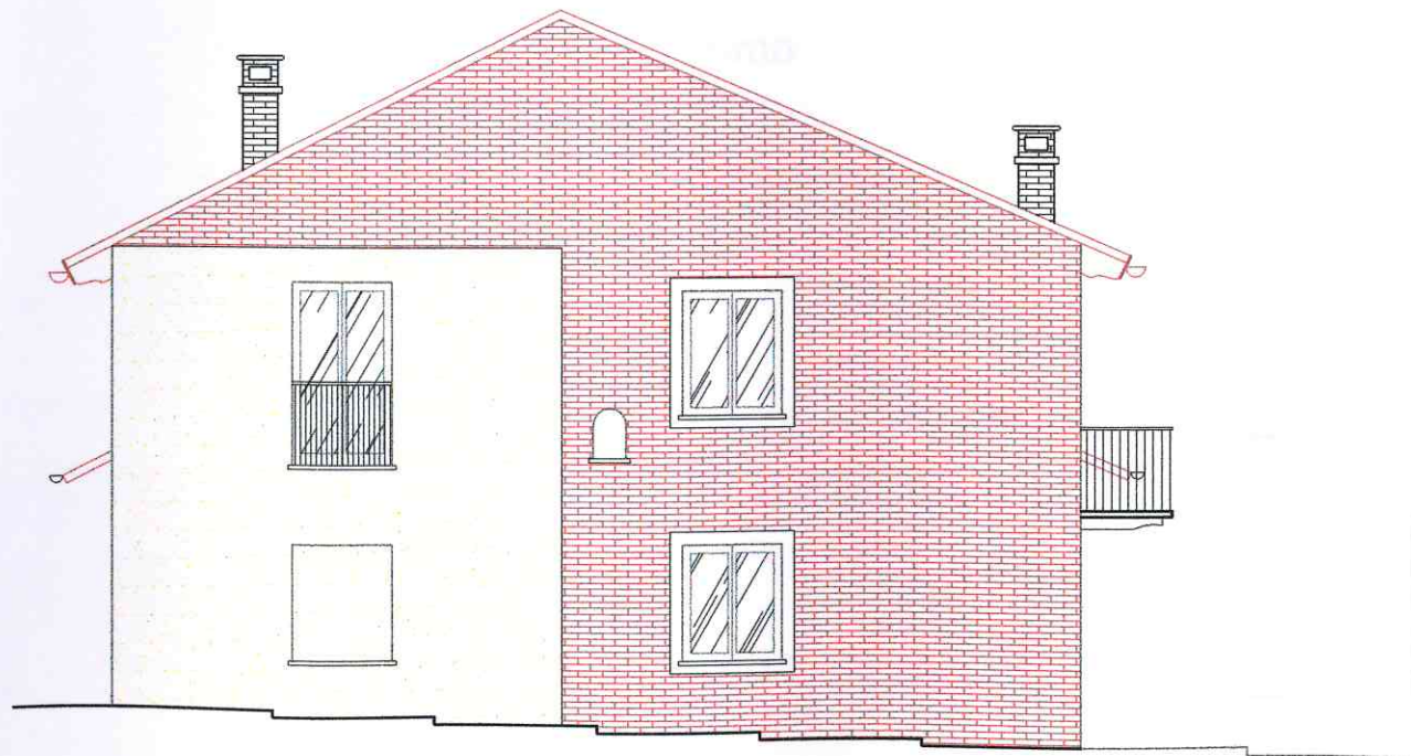
Prospetto ovest
