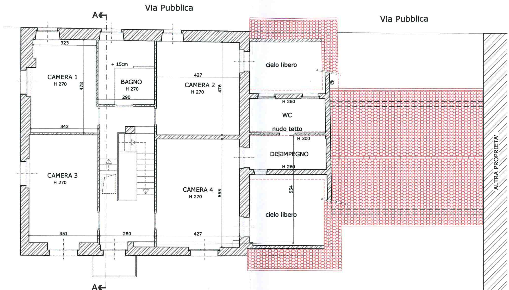
Planimetria del Piano Primo
