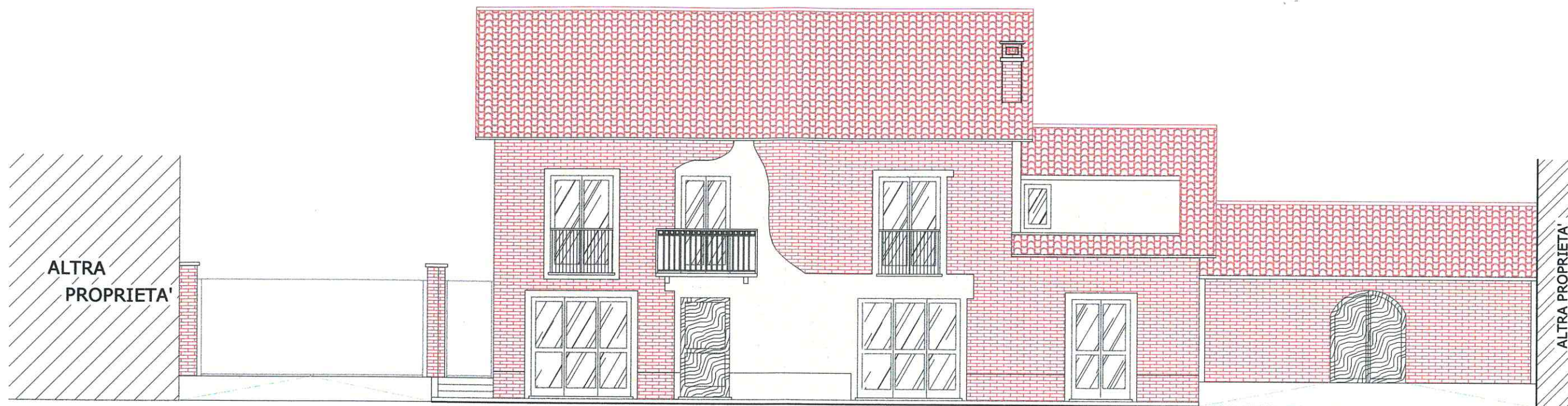
Prospetto sud
