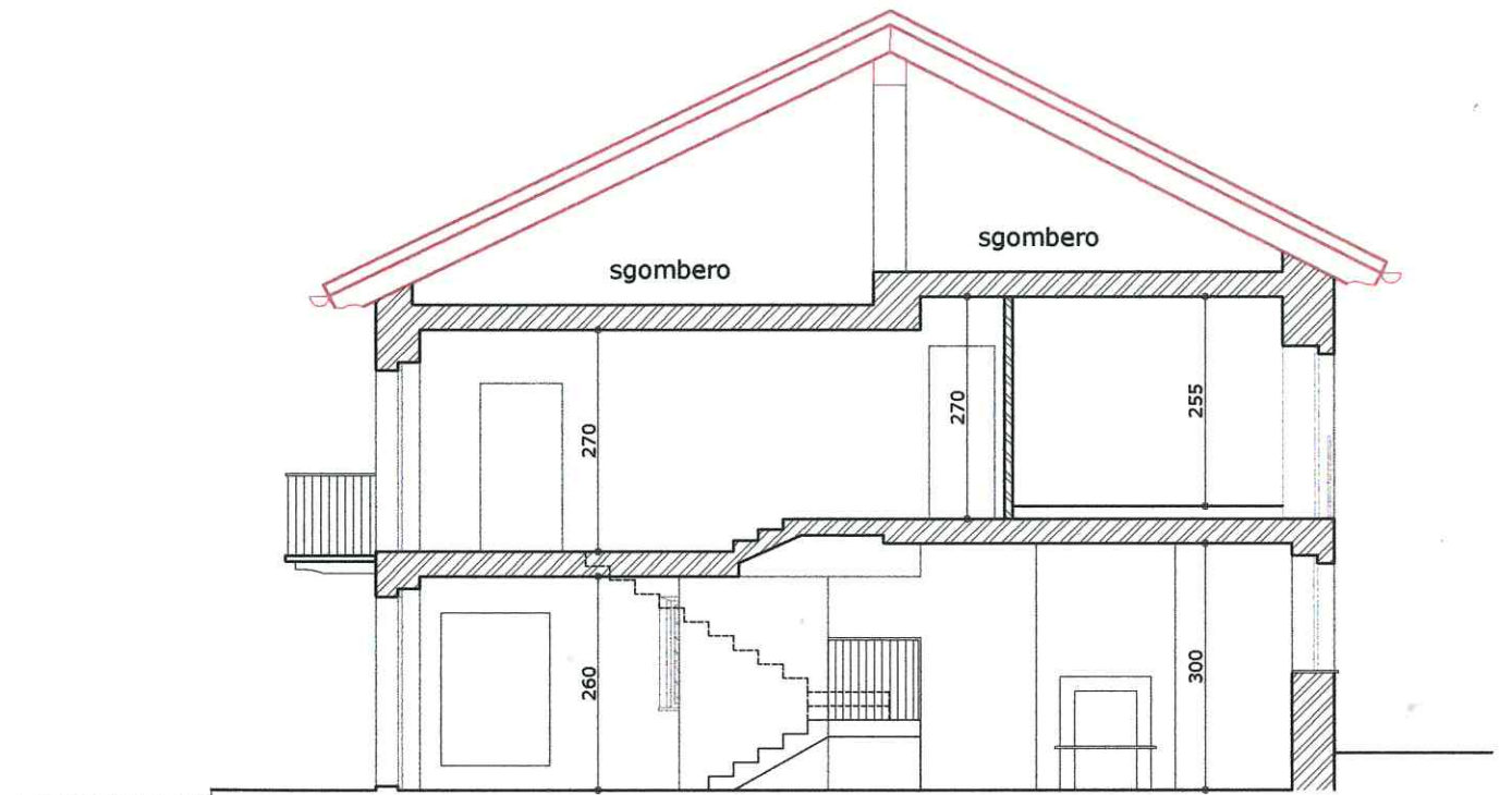
Sezione
