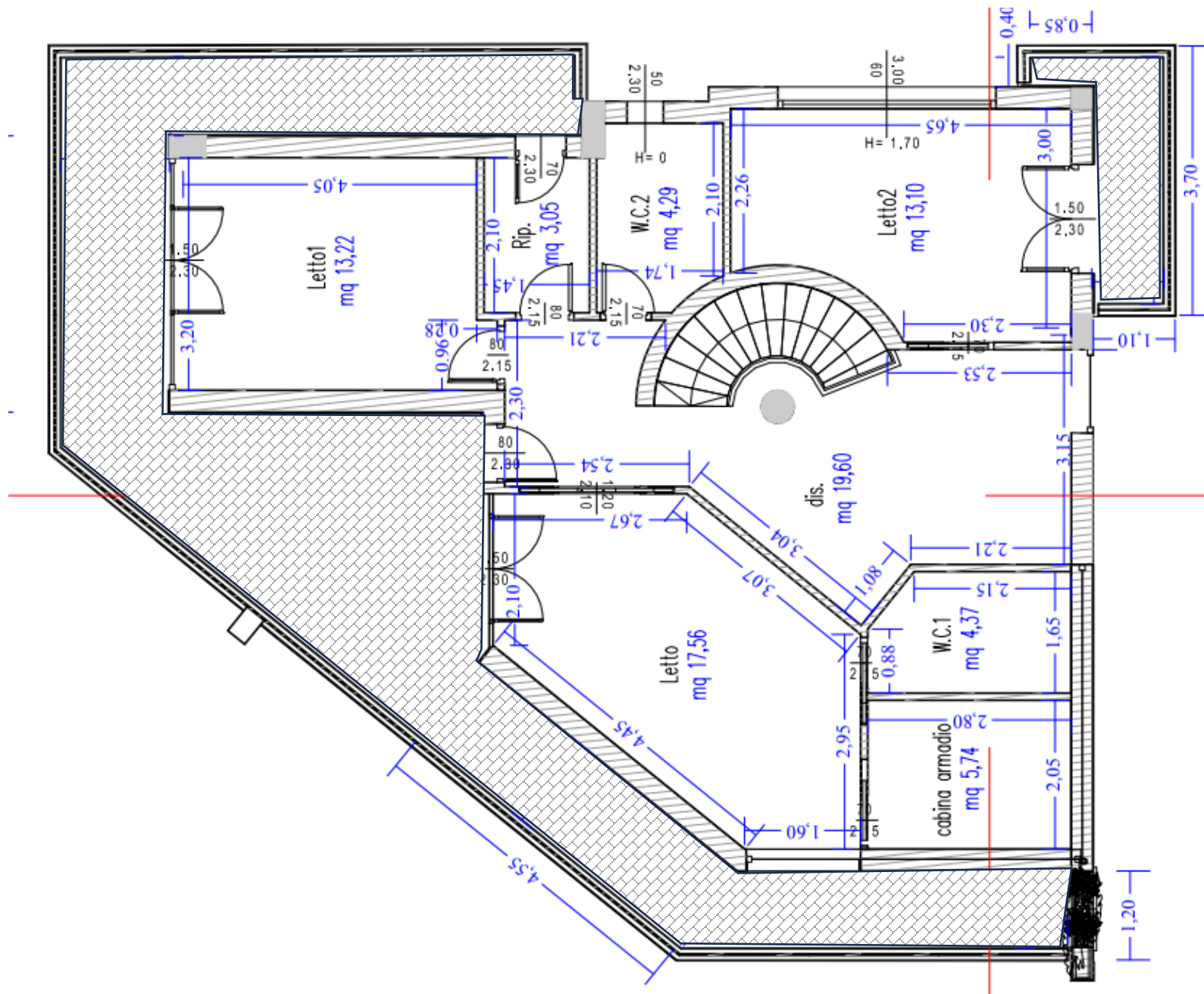
Piano Primo
