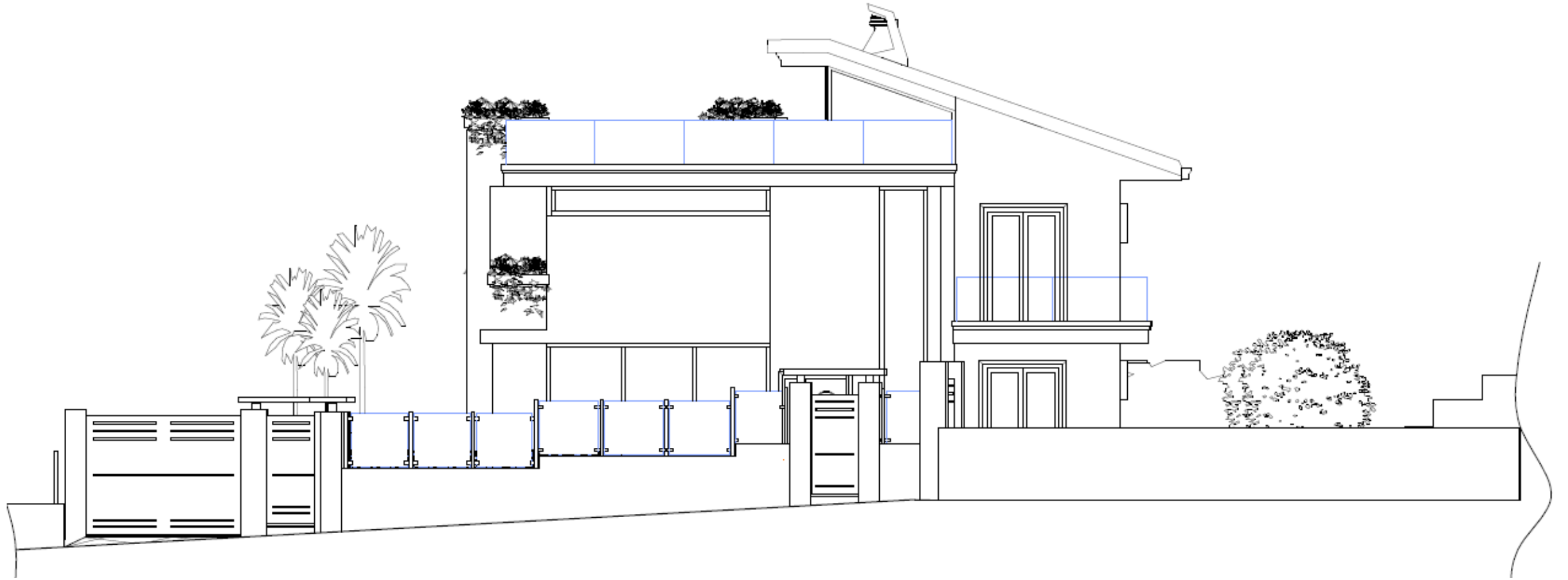
Prospetto Nord
