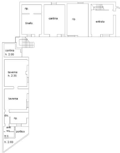
PIANO TERRA h. 2.85
