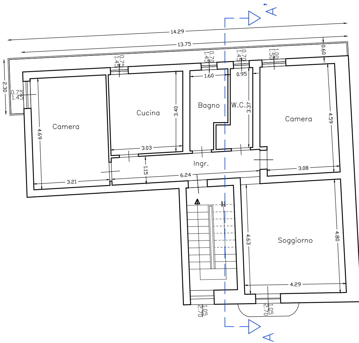
Pianta 1° piano scala 1:100
