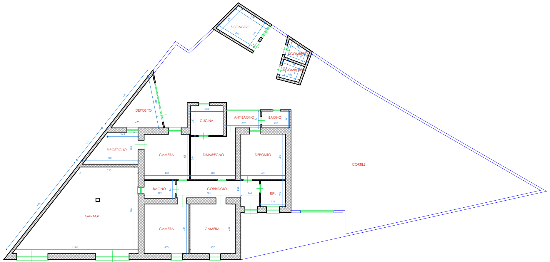
PIANTA STATO ATTUALE scala 1:200
