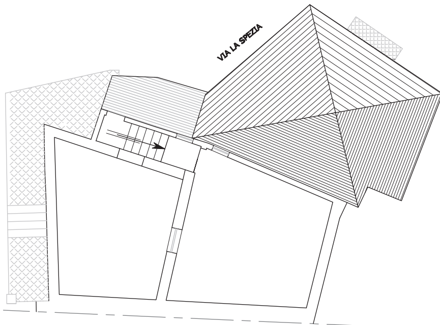
Pianta Sottotetto
