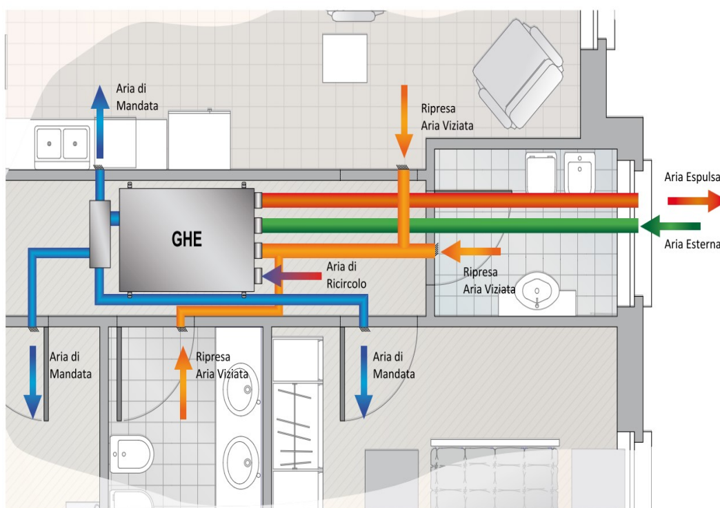
Installazione tipica
