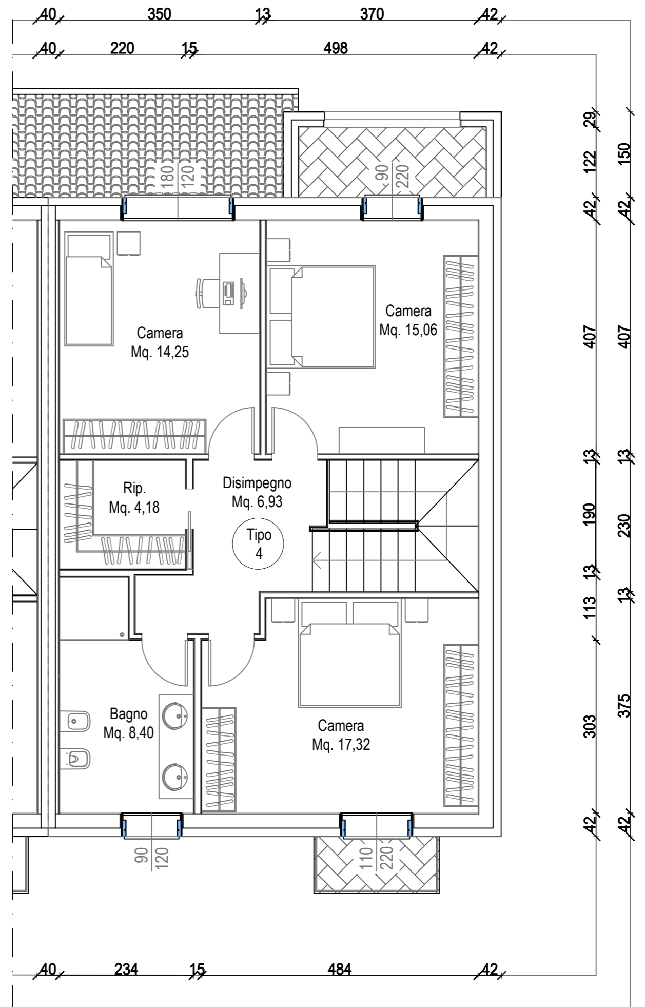
PIANTA PIANO PRIMO Unità Tipo 4
