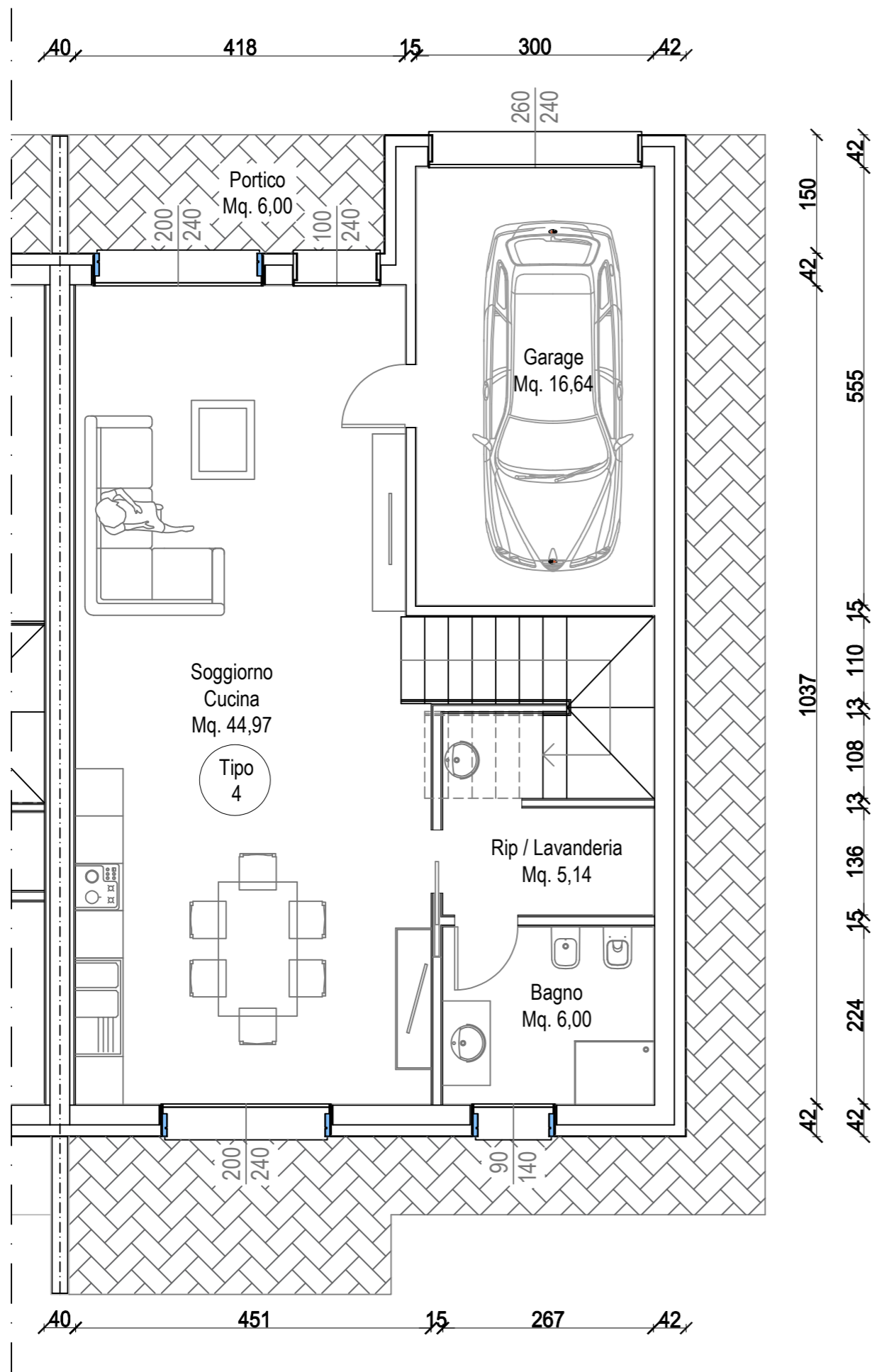
PIANTA PIANO TERRA Unità Tipo 4
