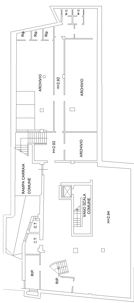
PIANO 1° SOTTOSTRADA
