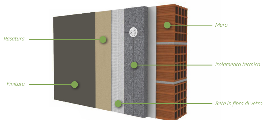
B2 - i _ Isolamento perimetrale a cappotto
