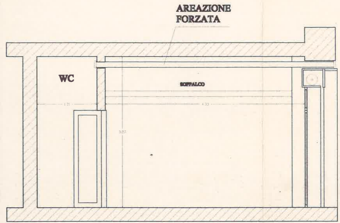
SEZIONE B-B SC. 1:50
