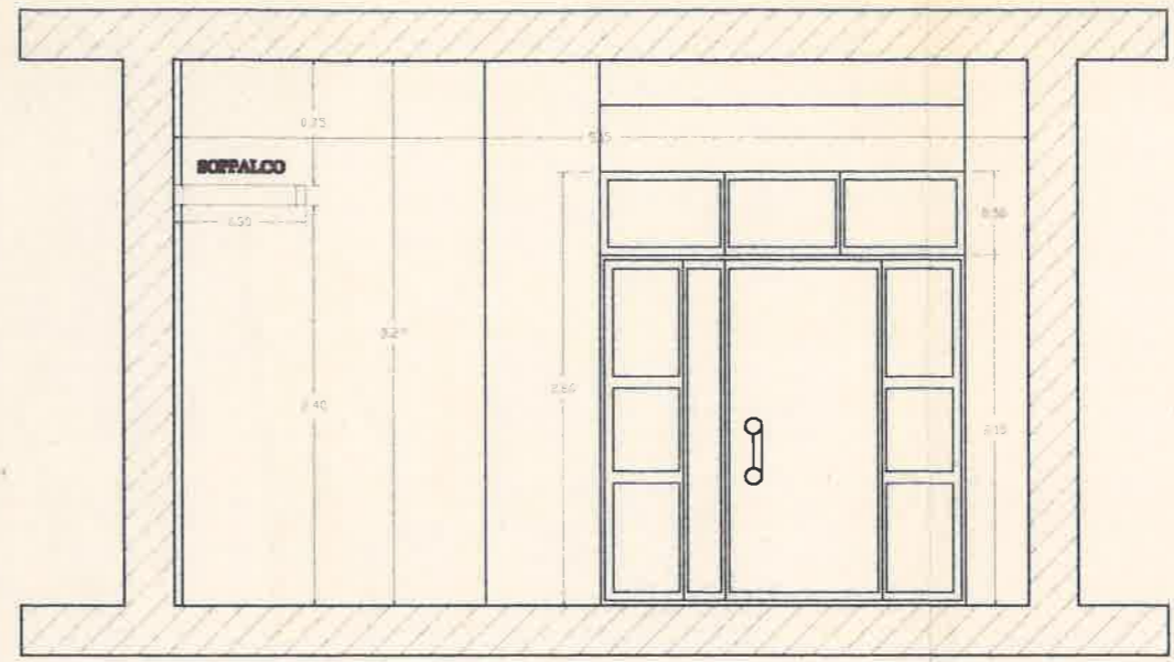
SEZIONE A-A SC. 1:50
