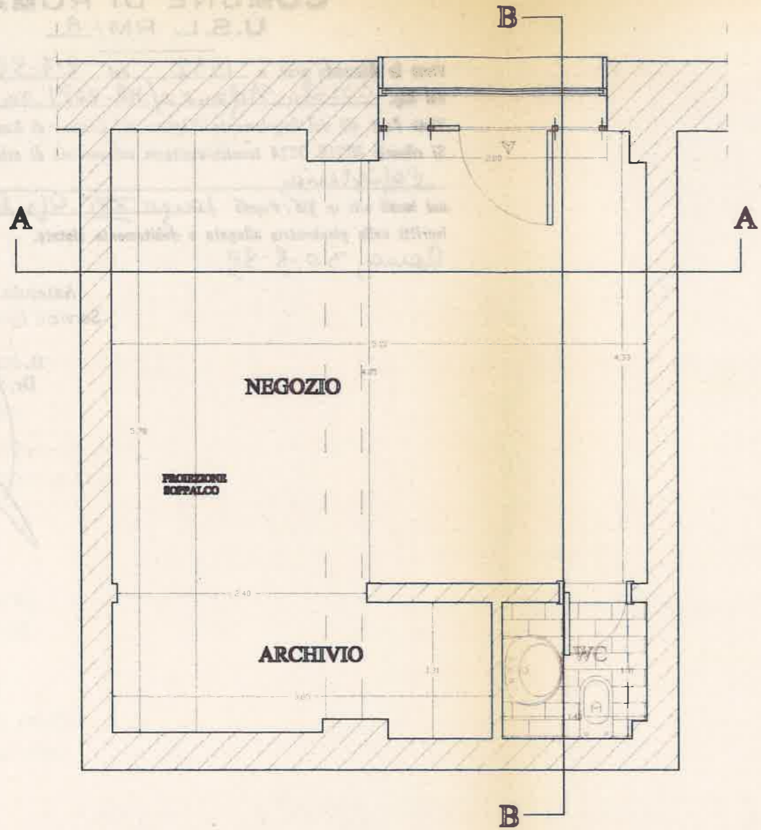
PIANTA P. TERRA SC. 1:50
