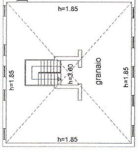
PIANTA PIANO SOTTOTETTO
