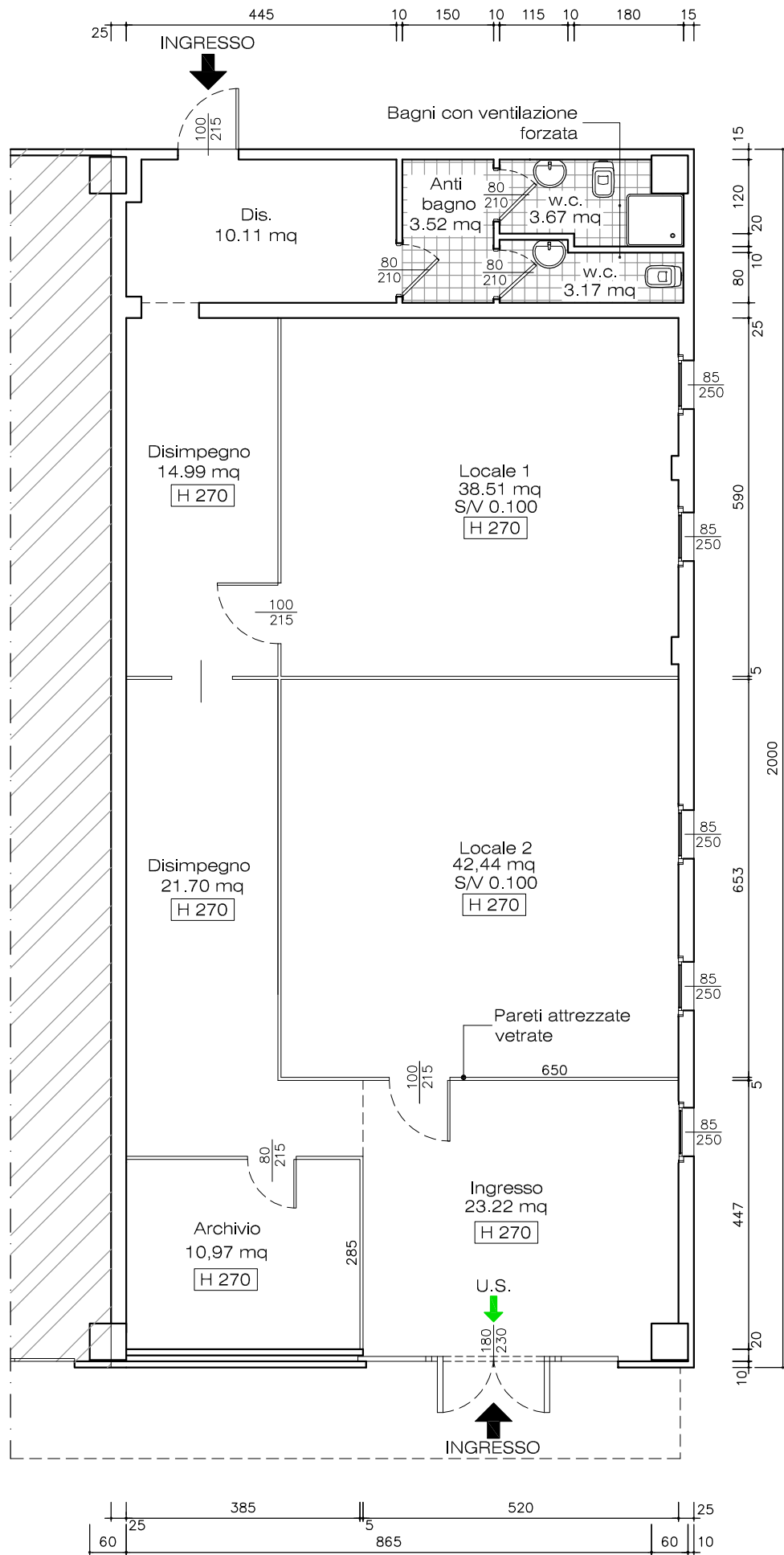
PIANTA Scala 1:100
